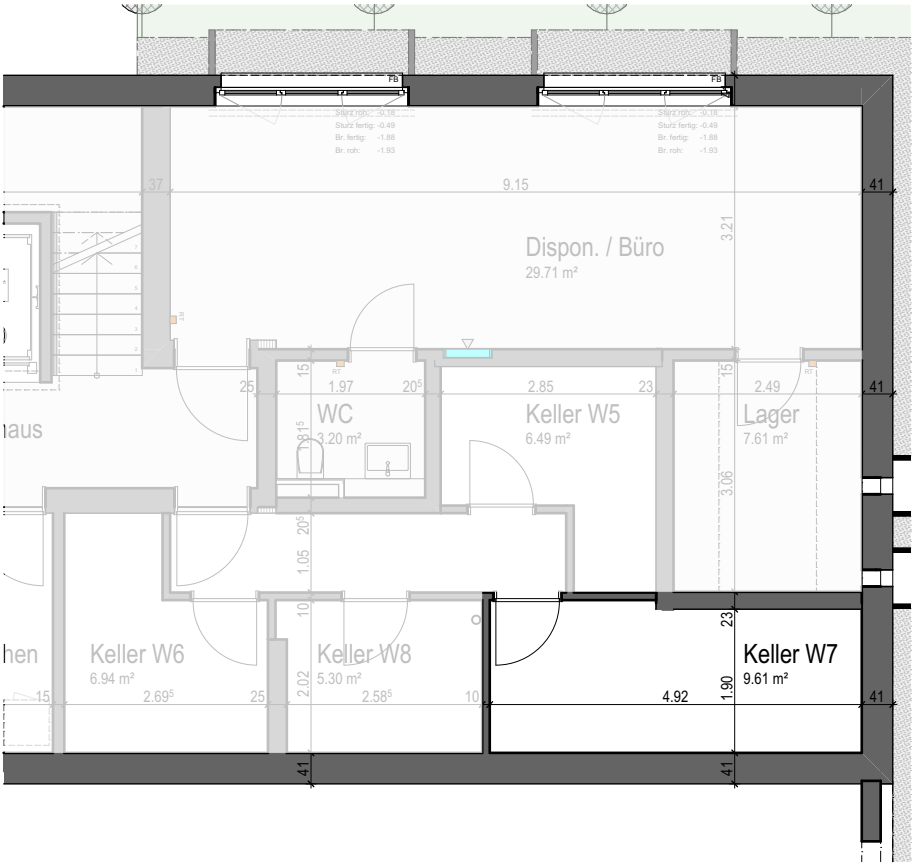
Untergeschoss Keller W7
