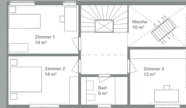
Obergeschoss Innenraumfläche OG ca. 69.3 m 2
