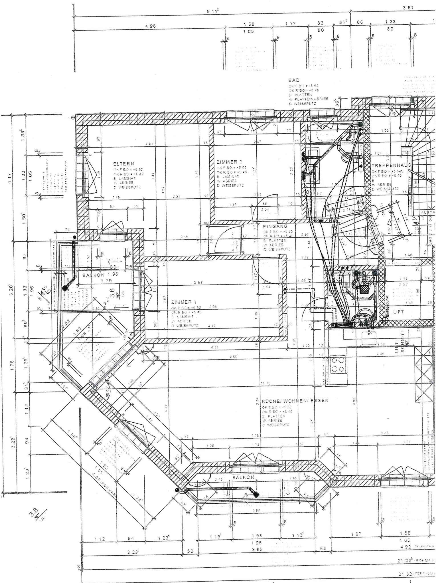
2. OBERGESCHOSS 1:50
