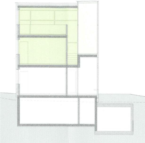
Querschnitt
