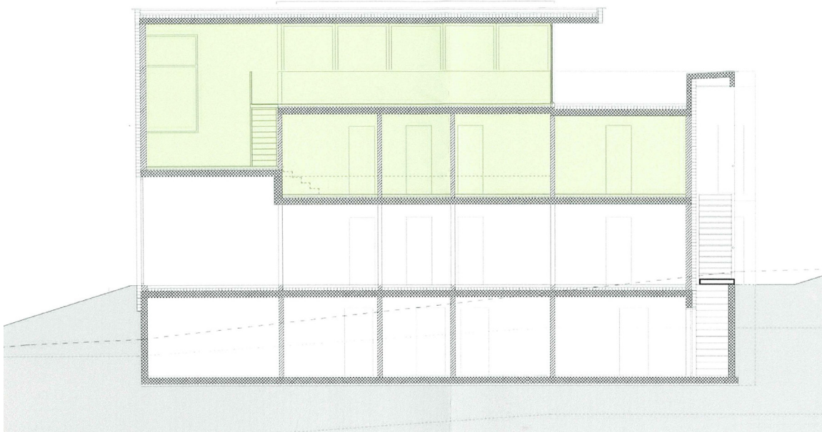
Längsschnitt
