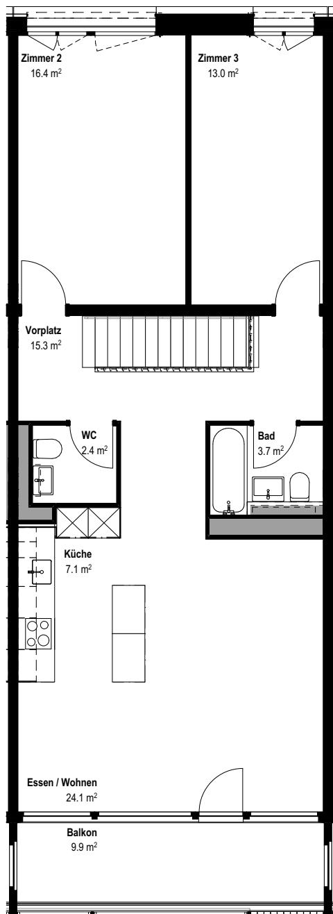
Wohnen 7.OG
