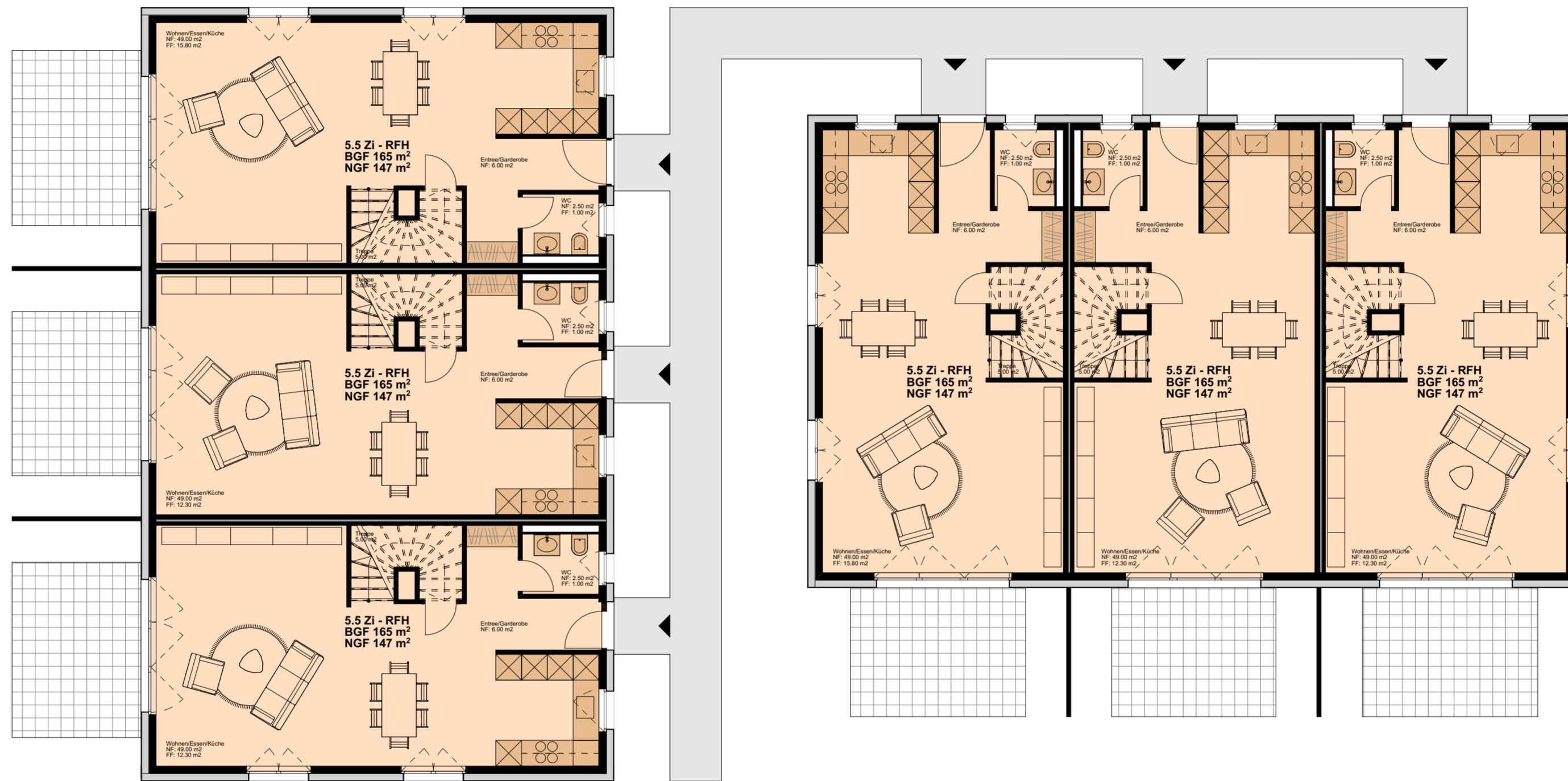
Grundriss Erdgeschoss
