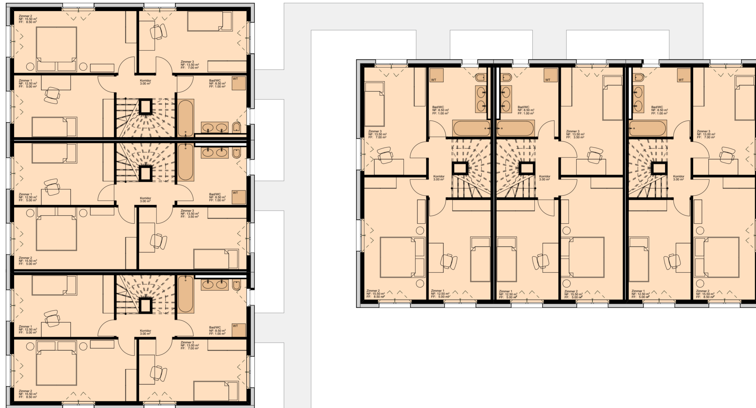
Grundriss Obergeschoss
