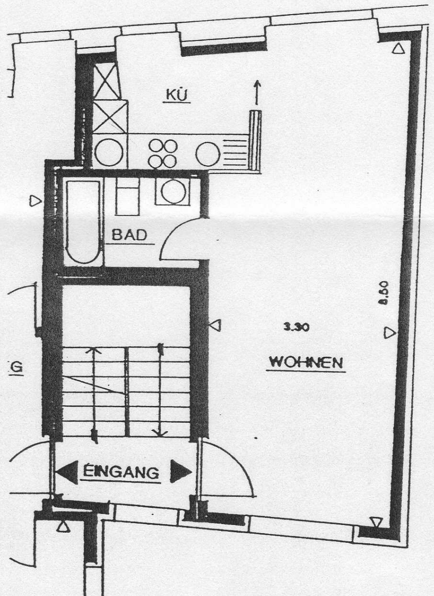
Grundriss 2./3. Obergeschoss Mst. 1:100
