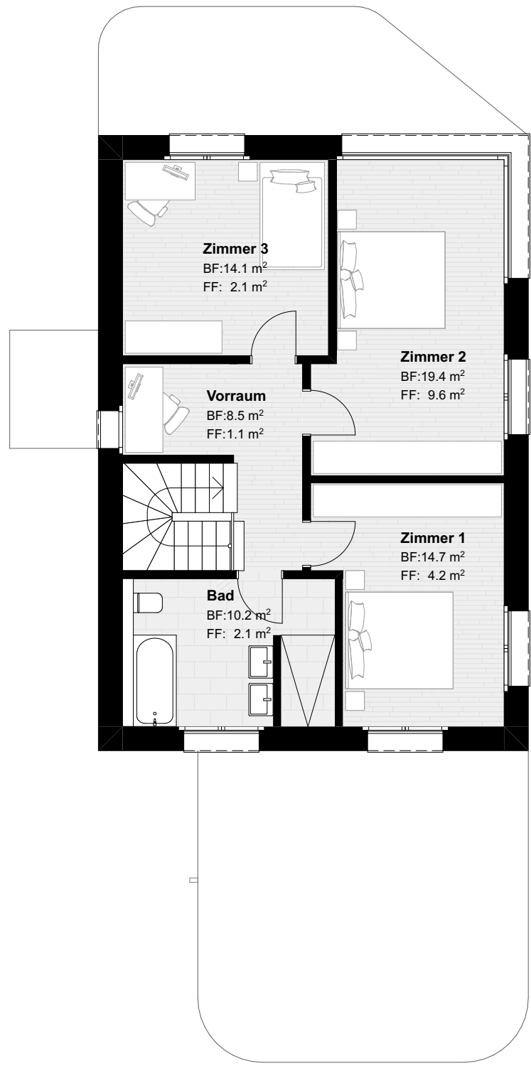
Obergeschoss
