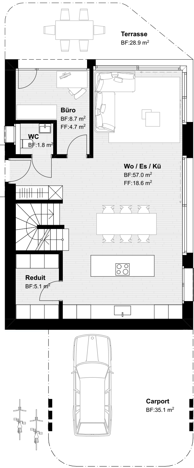
Erdgeschoss
