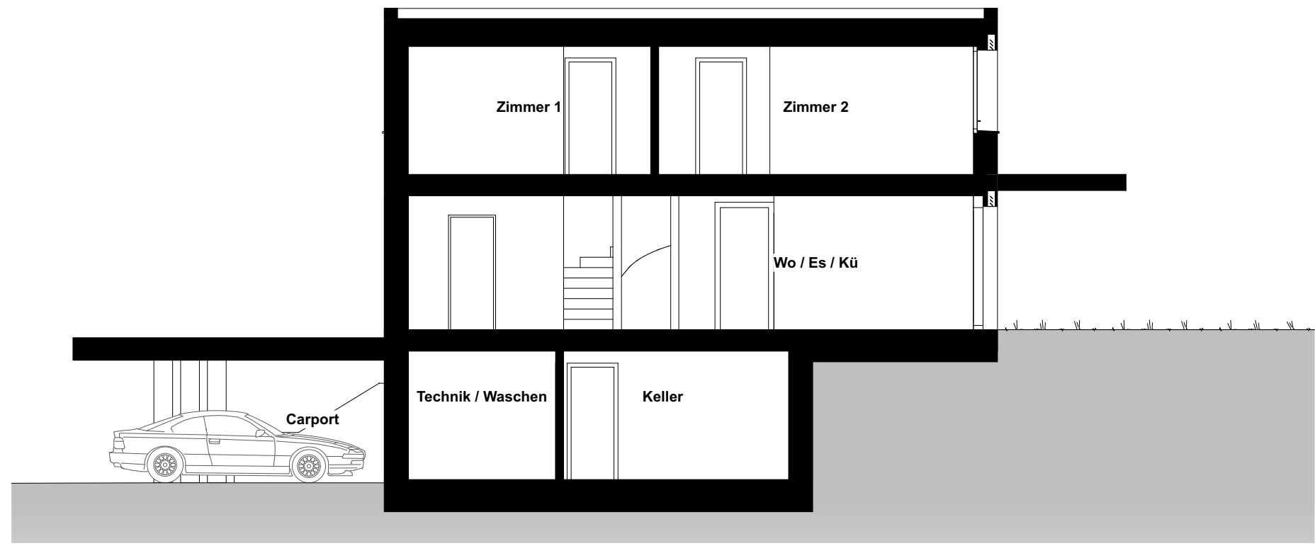
Schnitt Haus A
