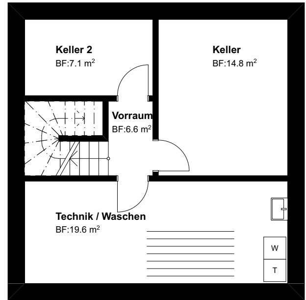
Untergeschoss
