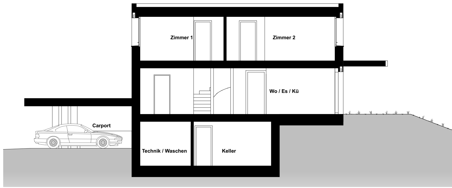
Schnitt Haus B
