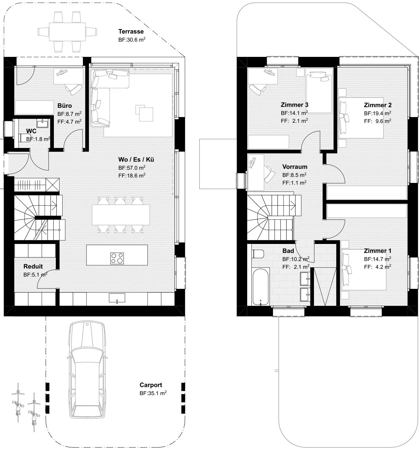
Erdgeschoss
