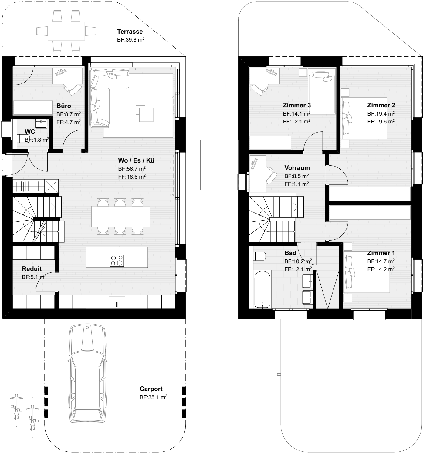
Erdgeschoss
