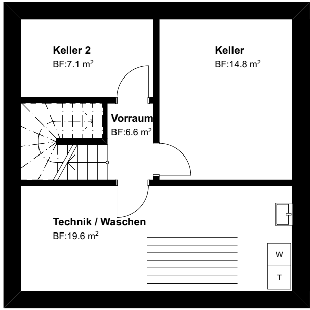
Untergeschoss
