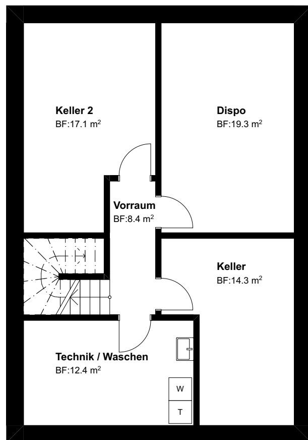
Untergeschoss
