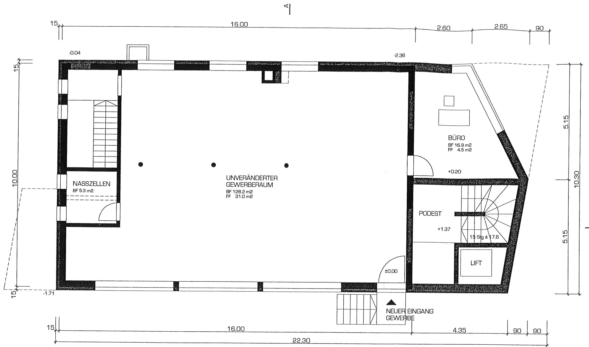
GRUNDRISS ERDGESCHOSS
