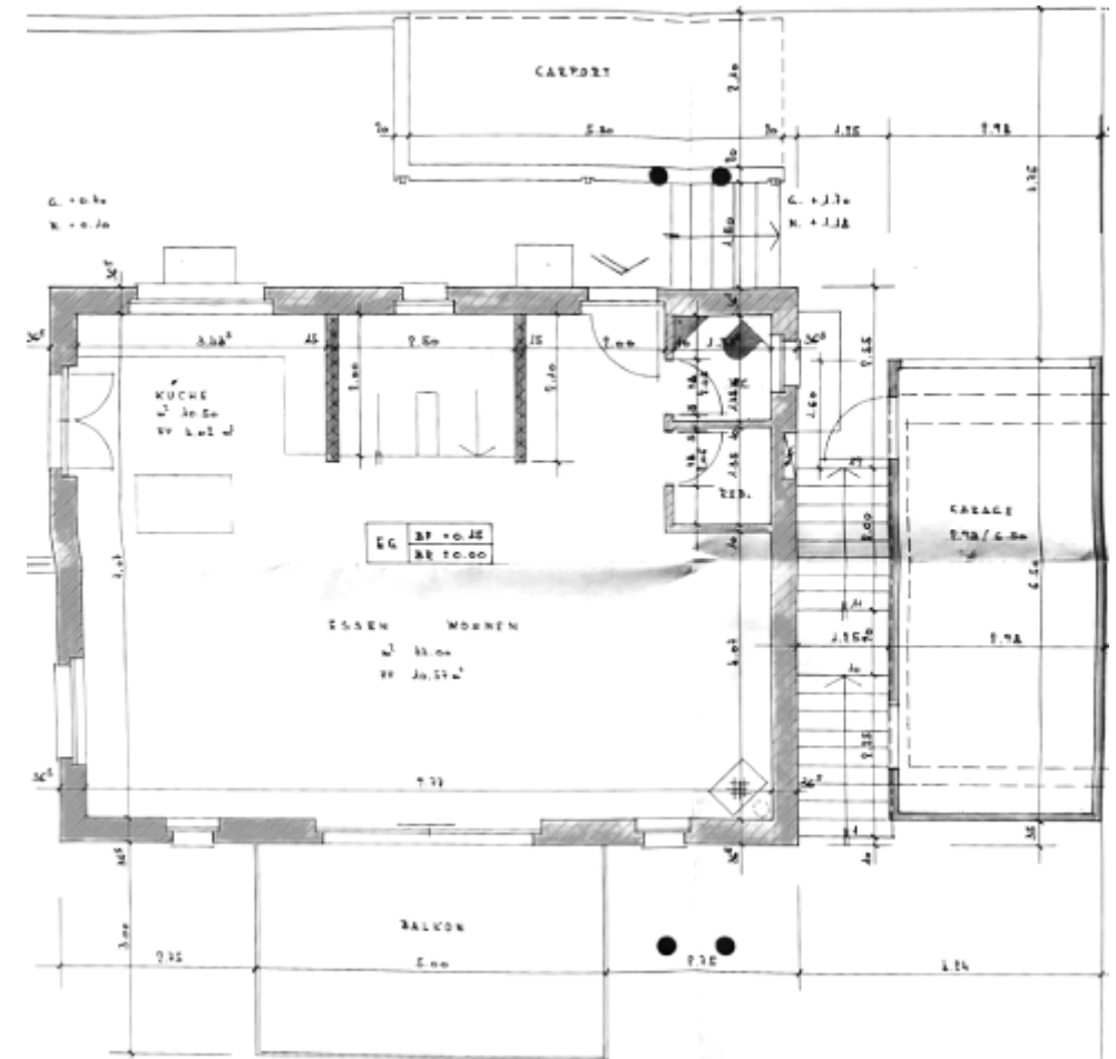
Grundriss Erdgeschoss
