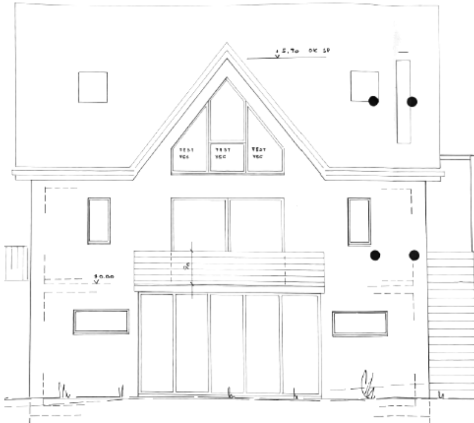
Nordfassade
