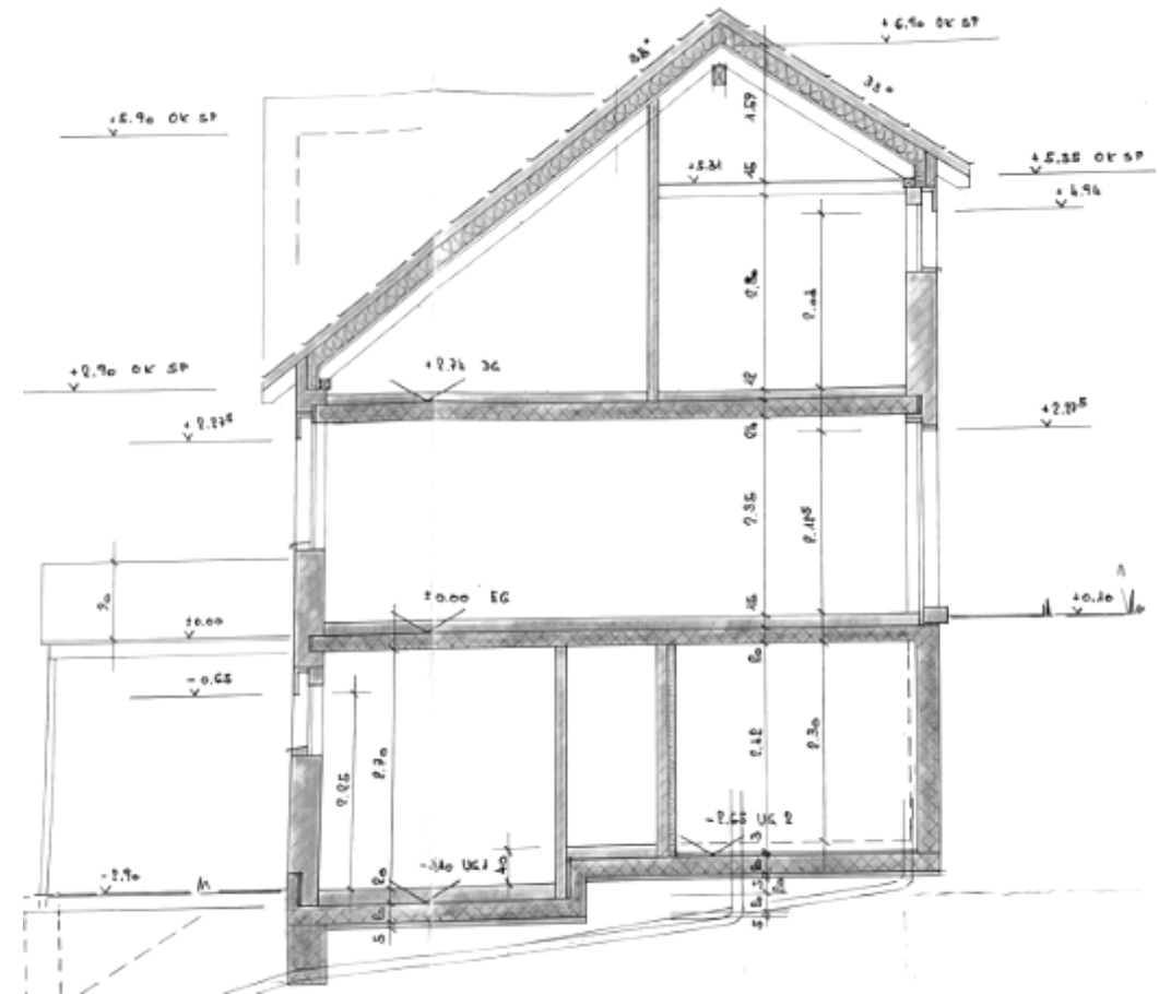
Querschnitt
