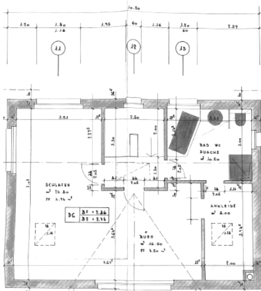
Grundriss Dachgeschoss
