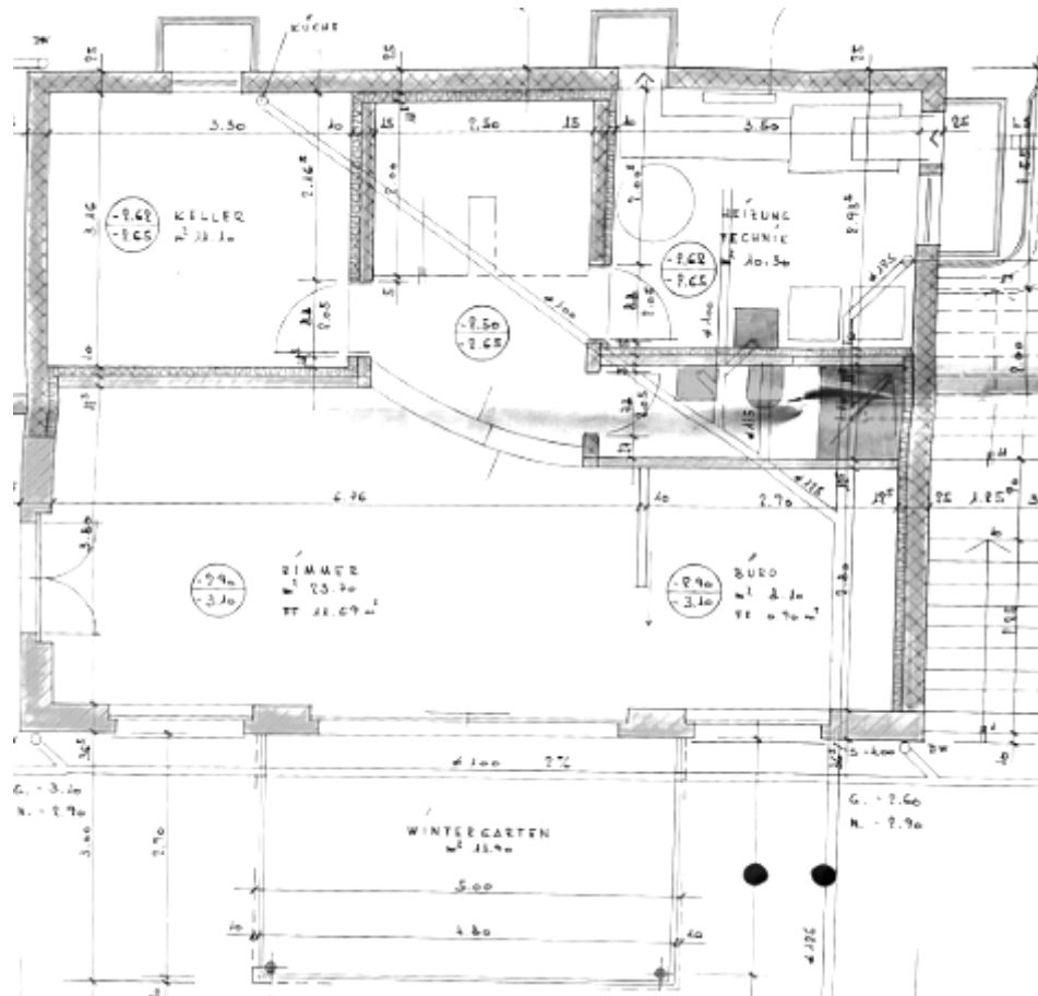
Grundriss Sockelgeschoss
