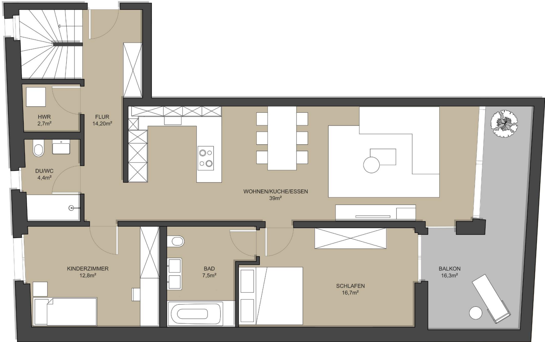
UNTERGESCHOSS 97,3m 2
