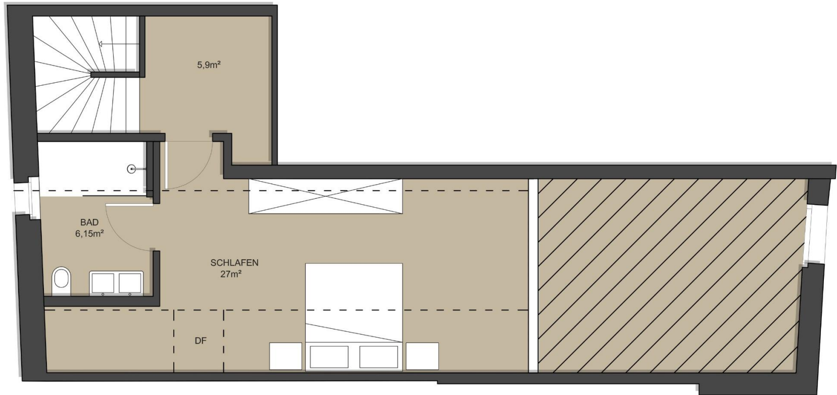
OBERGESCHOSS 39,10m 2
