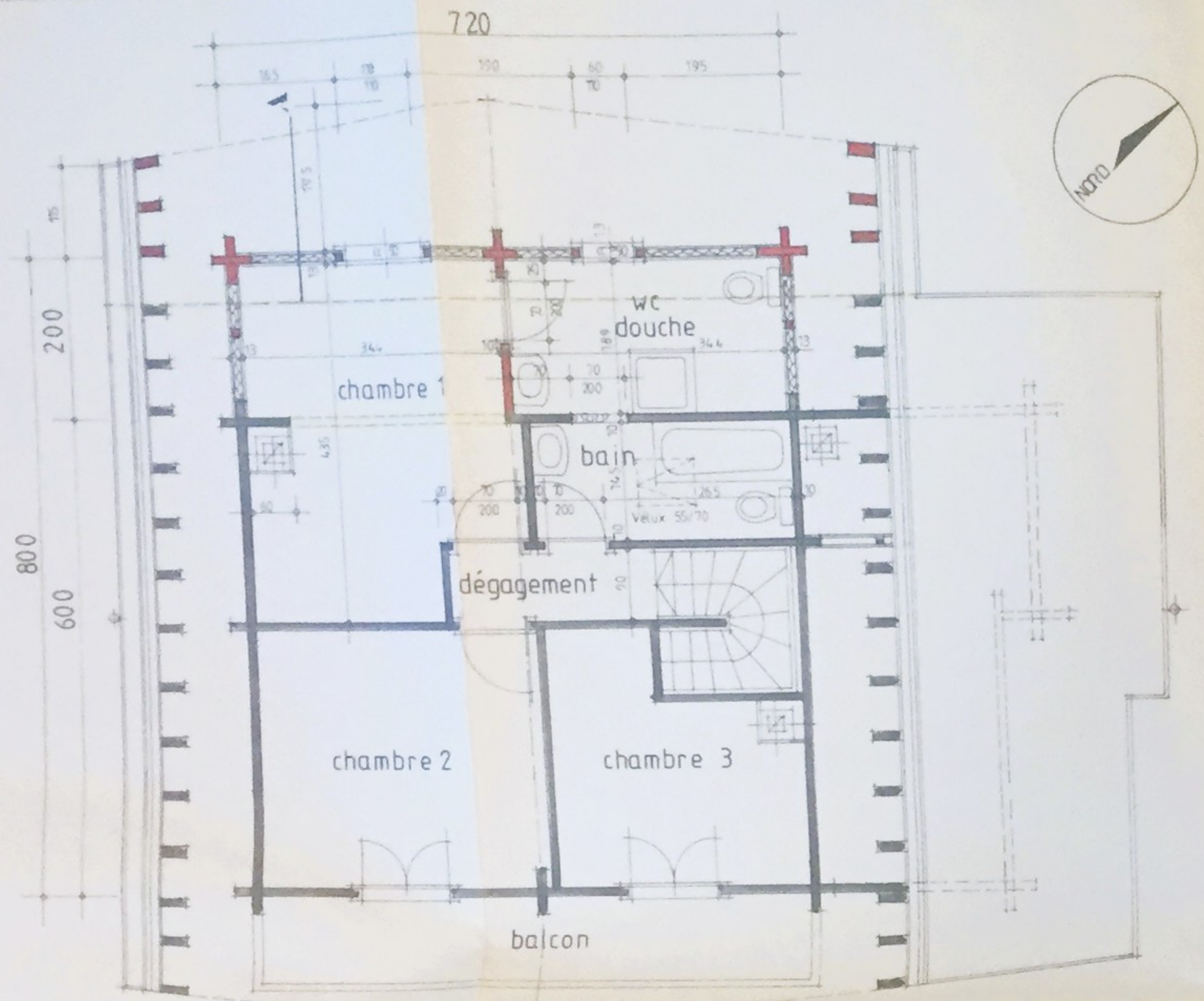
1 er ETAGE
