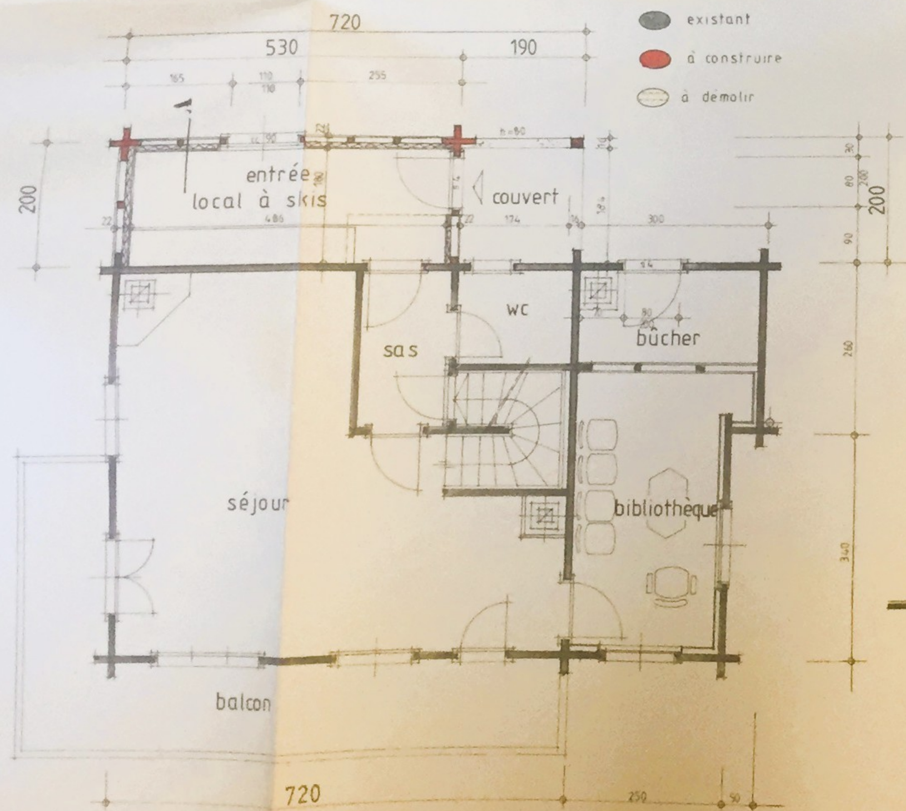
REZ-DE-CHAUSSEE
