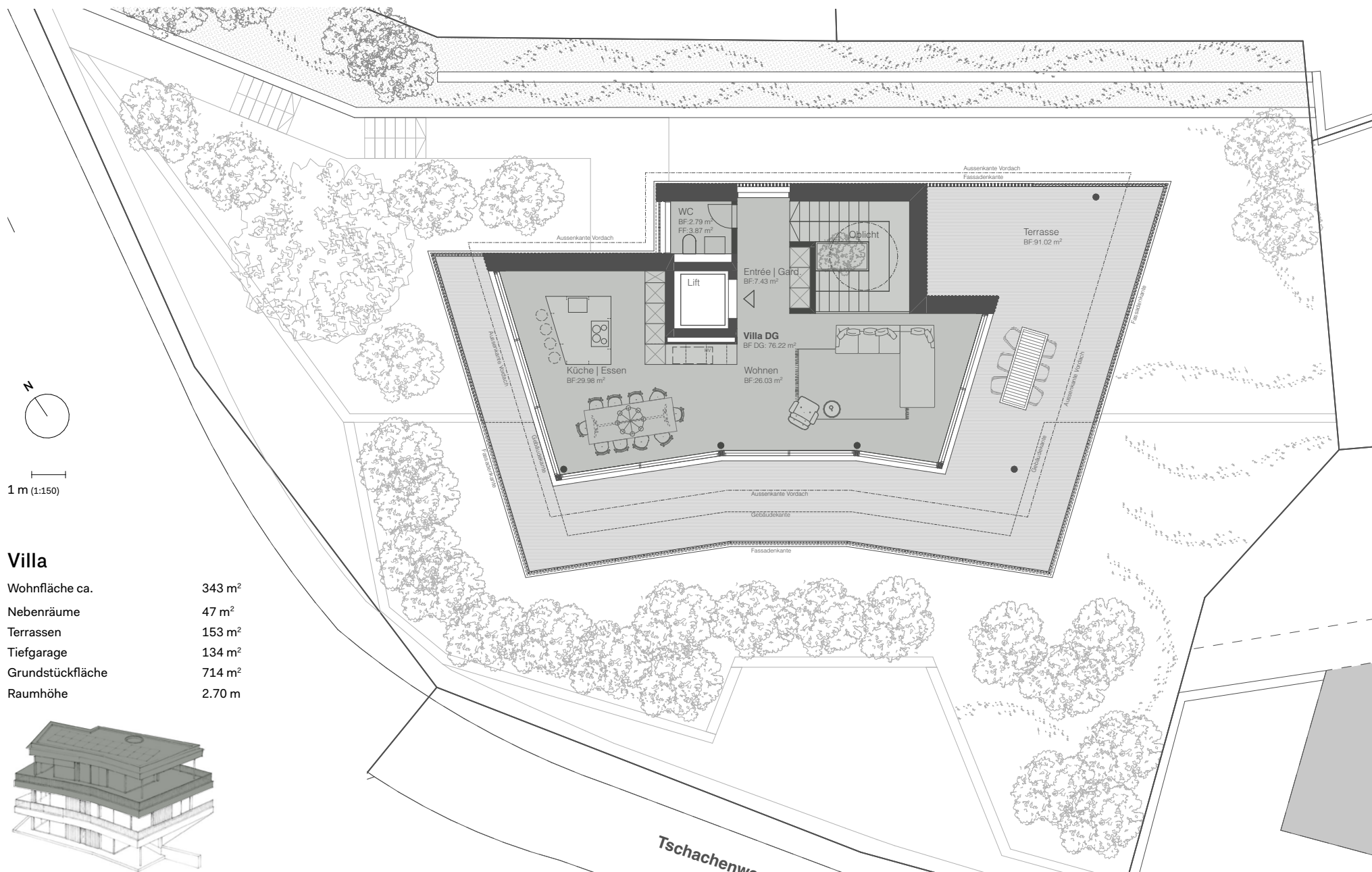
Grundriss Dachgeschoss
