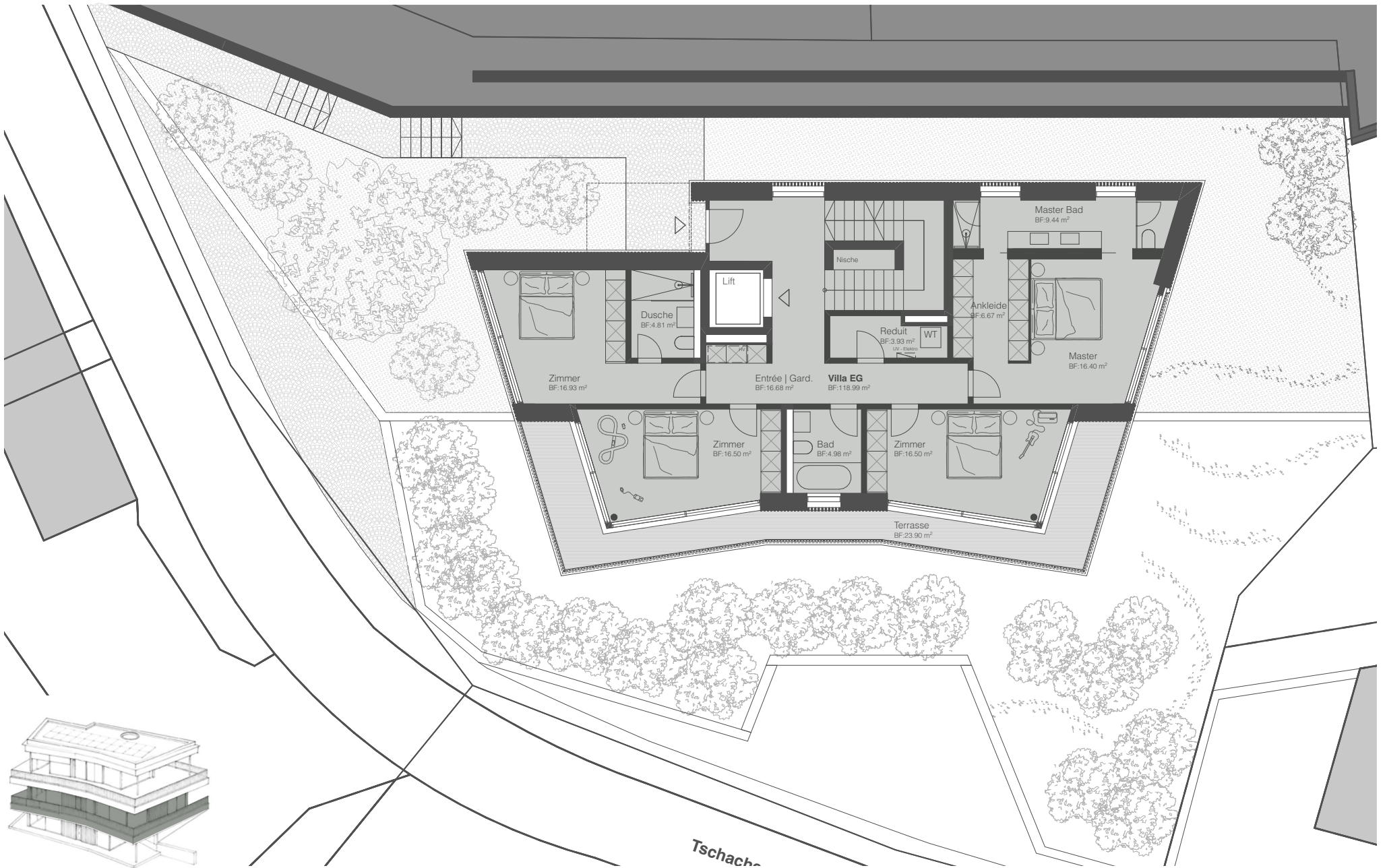
Grundriss Erdgeschoss
