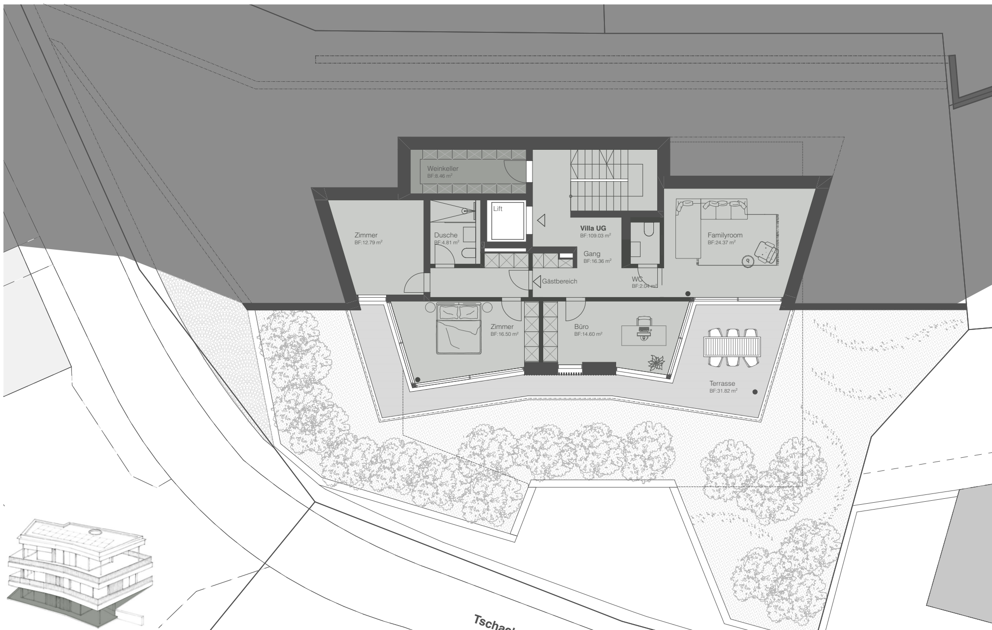
Grundriss Gartengeschoss
