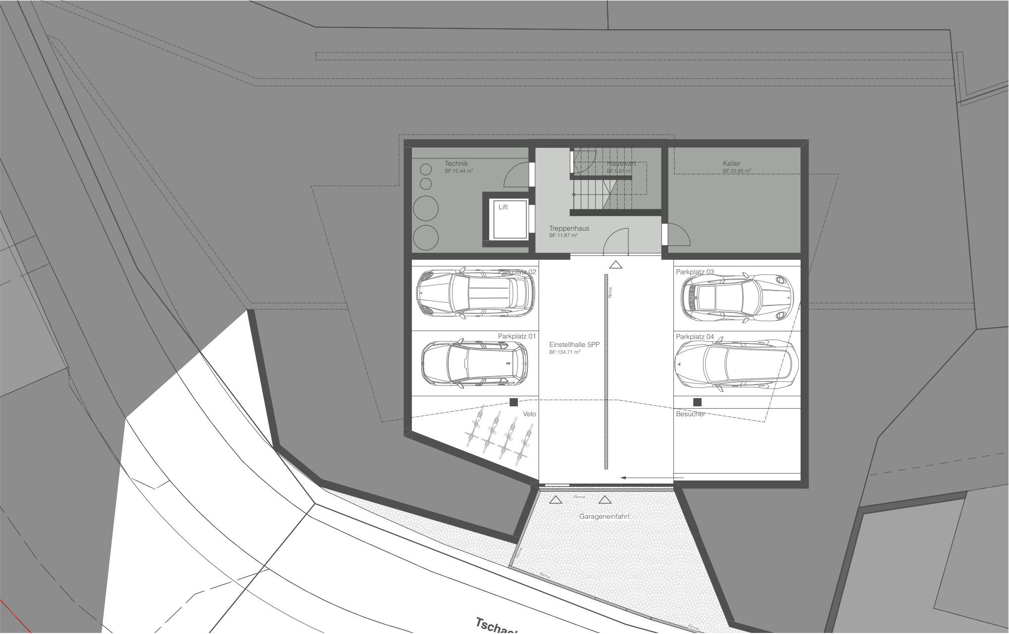
Grundriss Garagengeschoß
