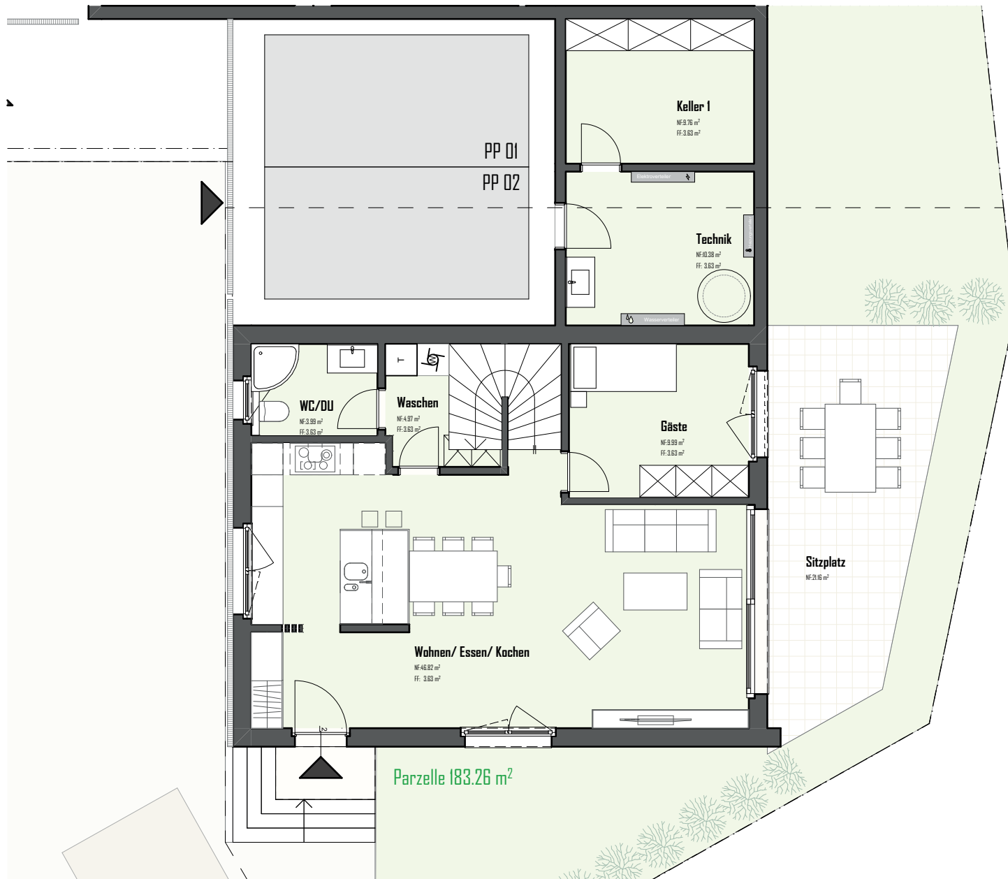
Erdgeschoss mit Keller, Haus 1
