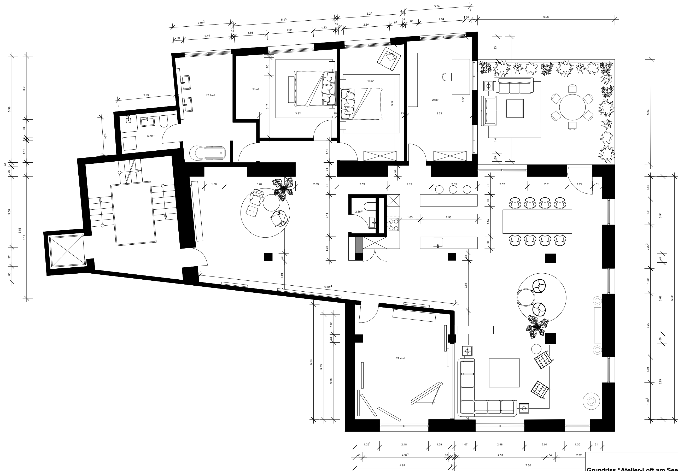
Grundriss "Atelier-Loft am See"
