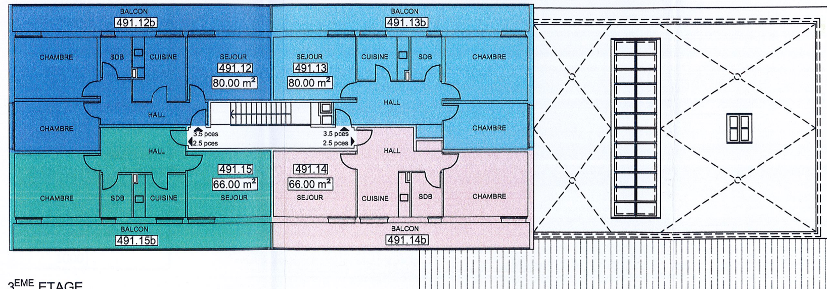
3 EME ETAGE
