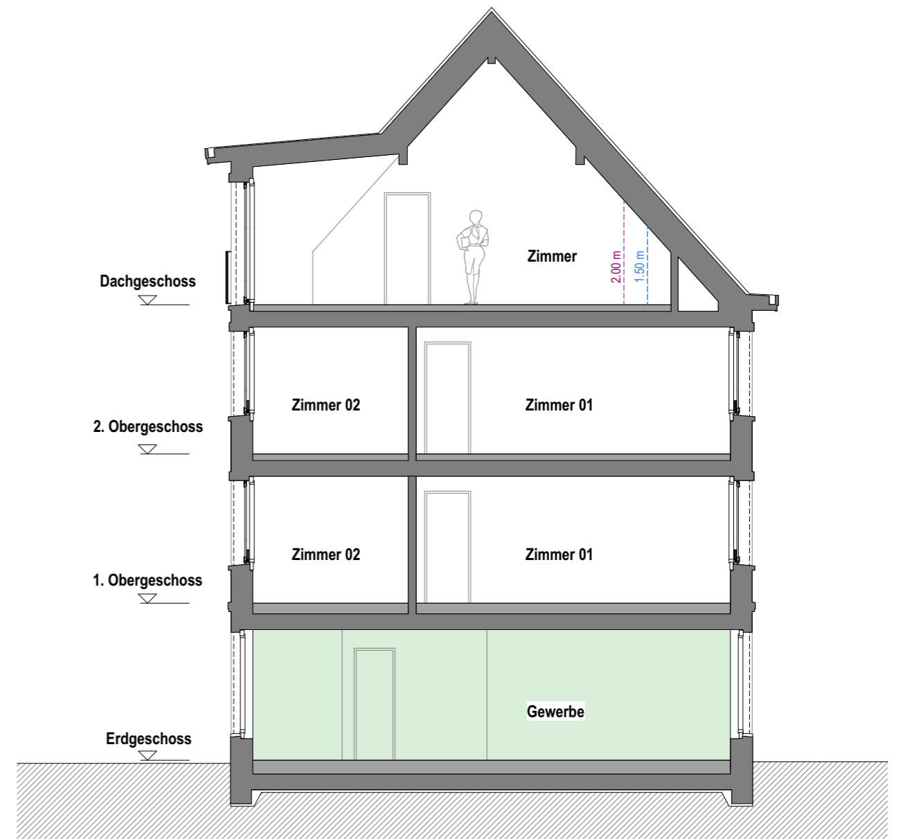
Querschnitt Mst. 1:100
