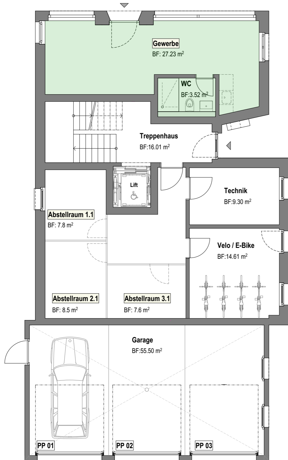
Erdgeschoss Mst. 1:100
