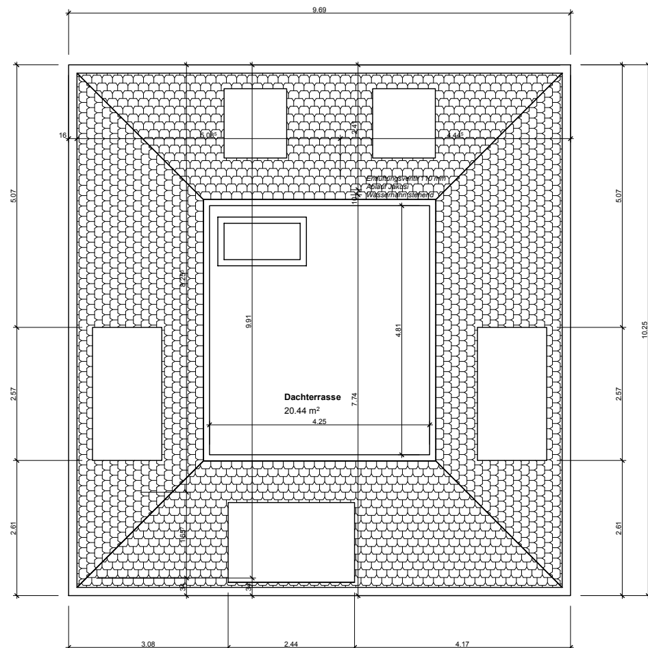
Dachaufsicht 1: 100
