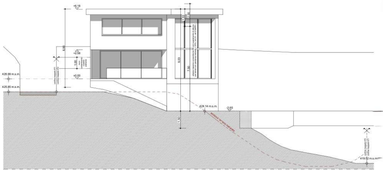
FACCIATA SUD
