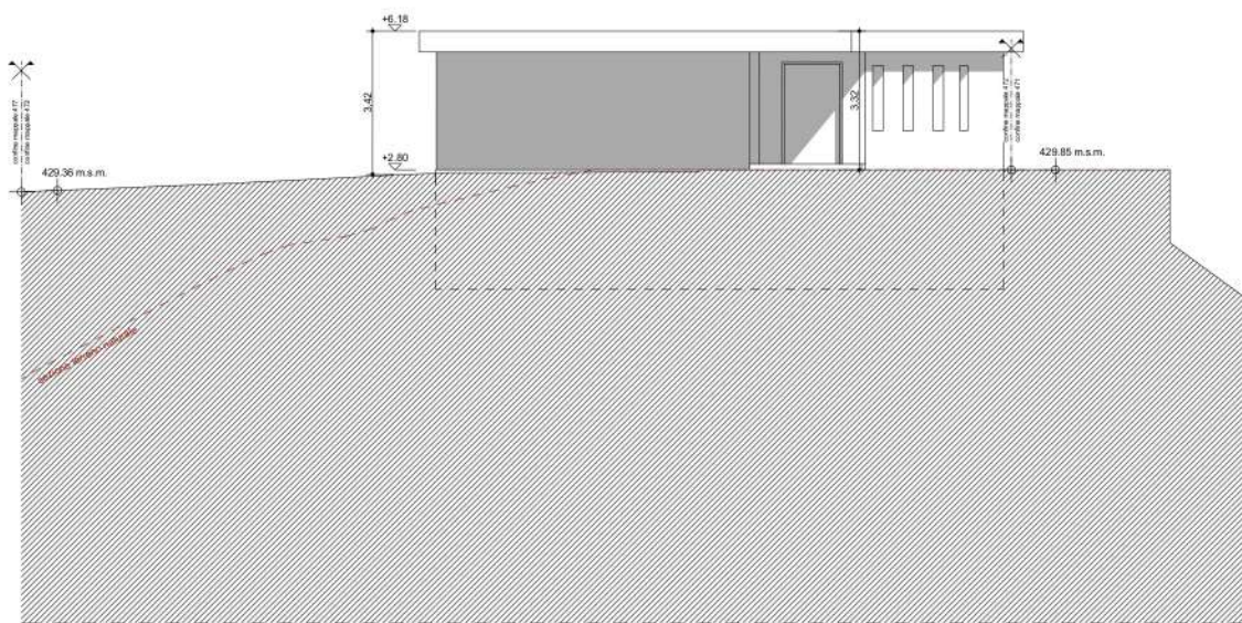
FACCIATA NORD
