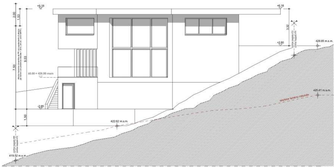
FACCIATA EST
