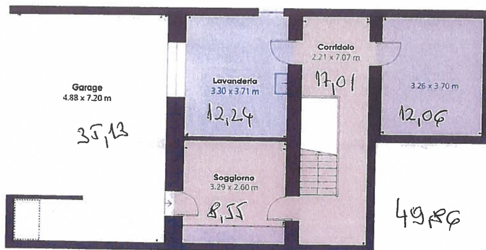
Seminterrato / Untergeschoss
