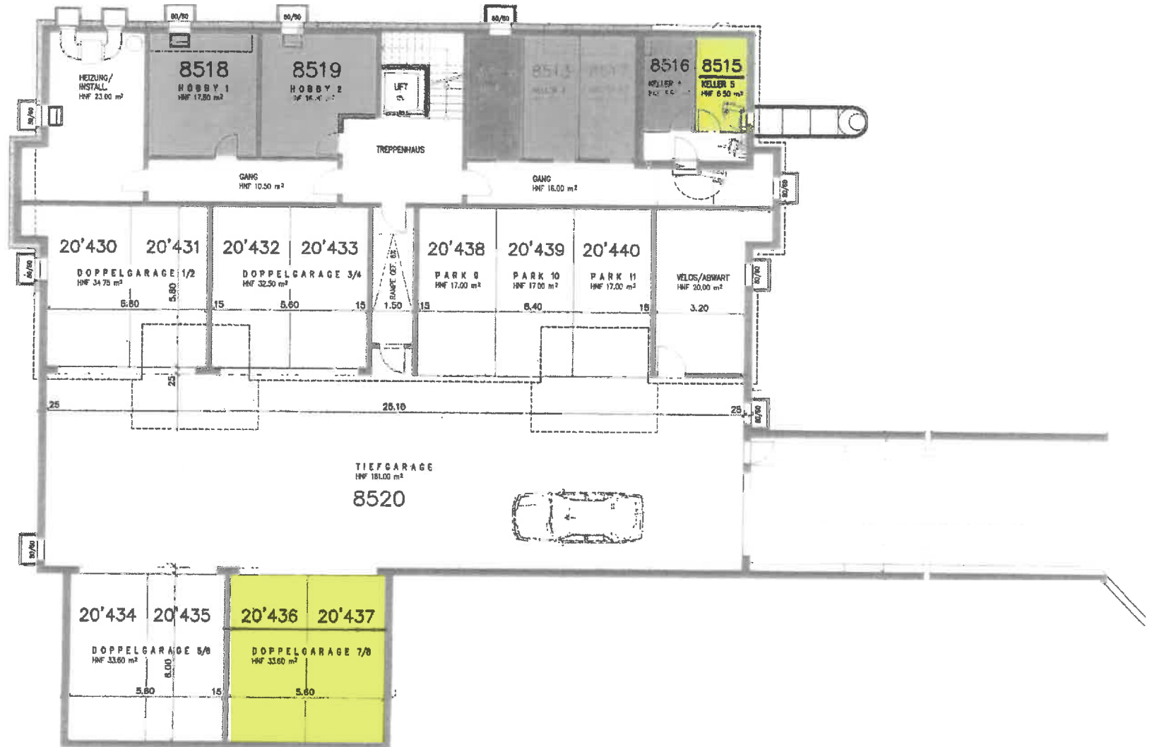
Grundriss Untergeschoss
