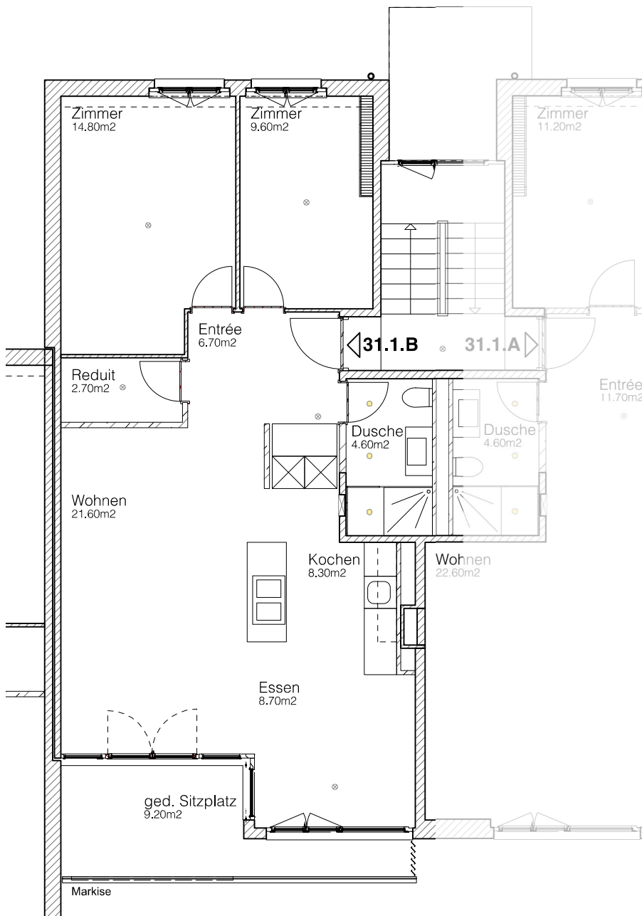
Grundriss Mst. 1:100
