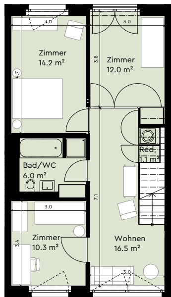
2. OBERGESCHOSS
