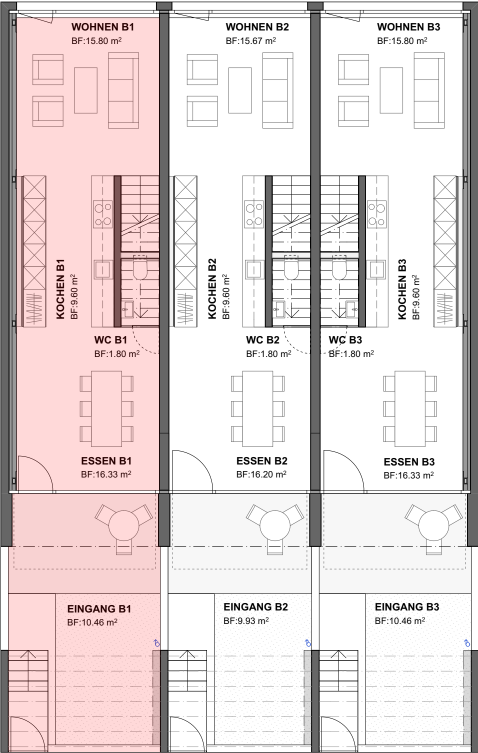
ERDGESCHOSS
