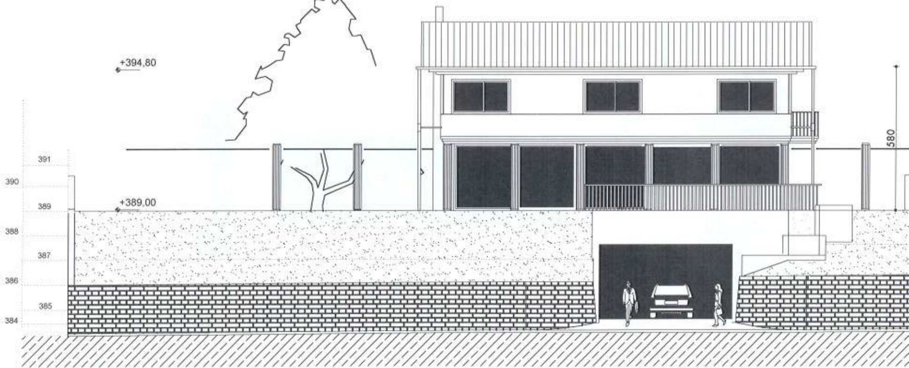
PROSPETTO SUD-EST
