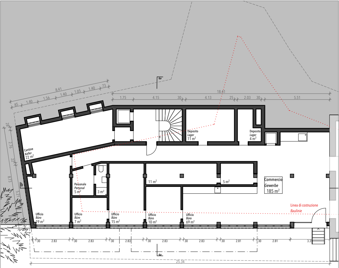
1. piano | 1. Obergeschoss
