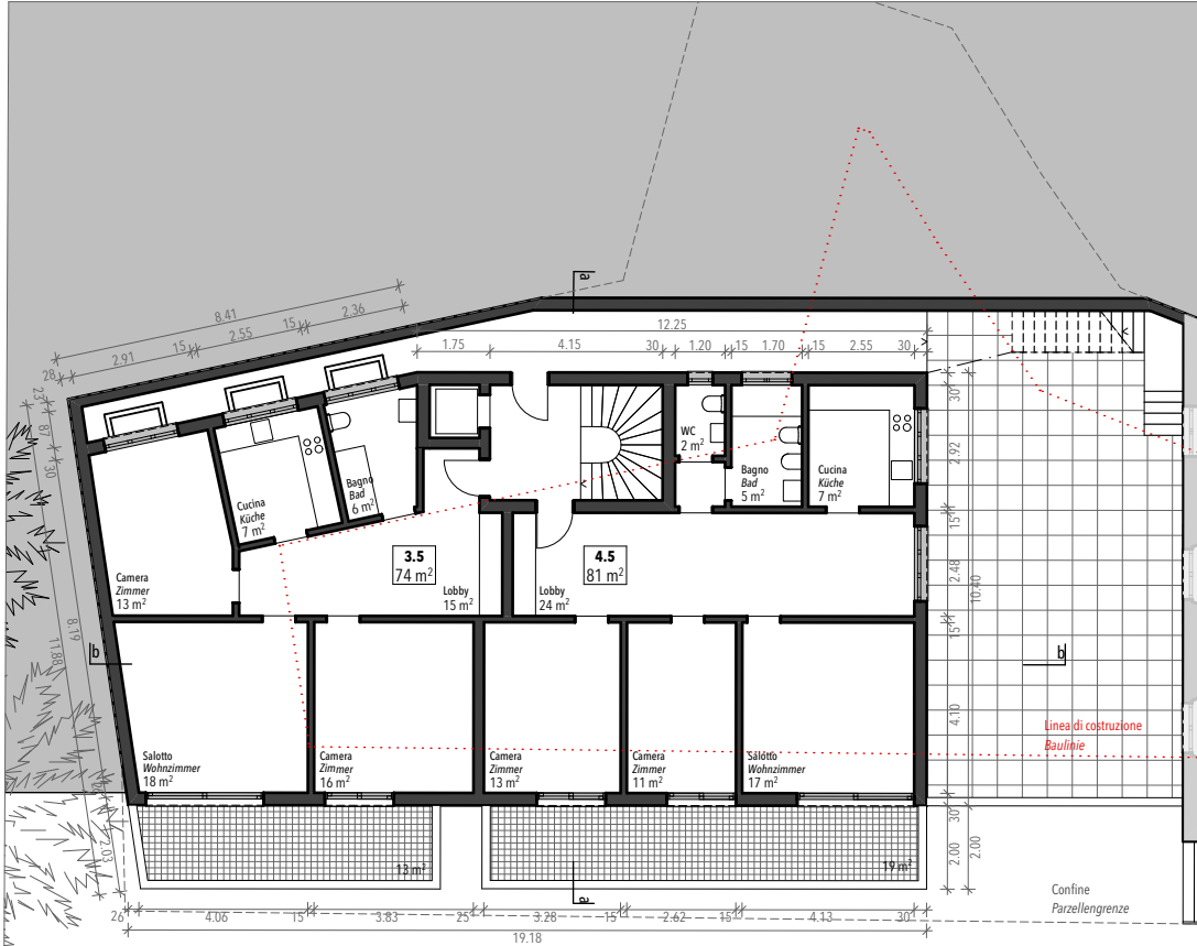
2. piano | 2. Obergeschoss
