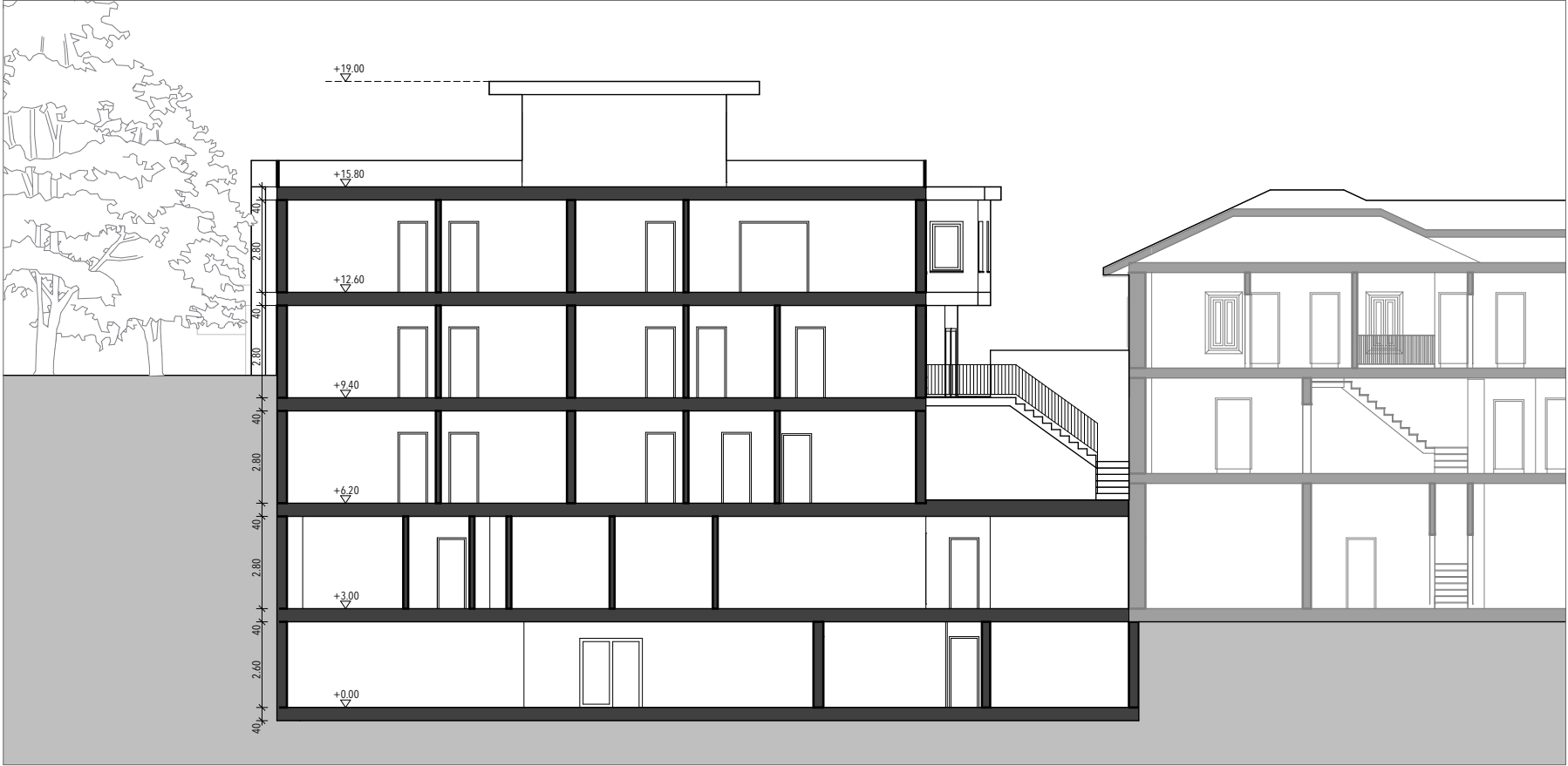
Sezione BB | Schnitt BB
