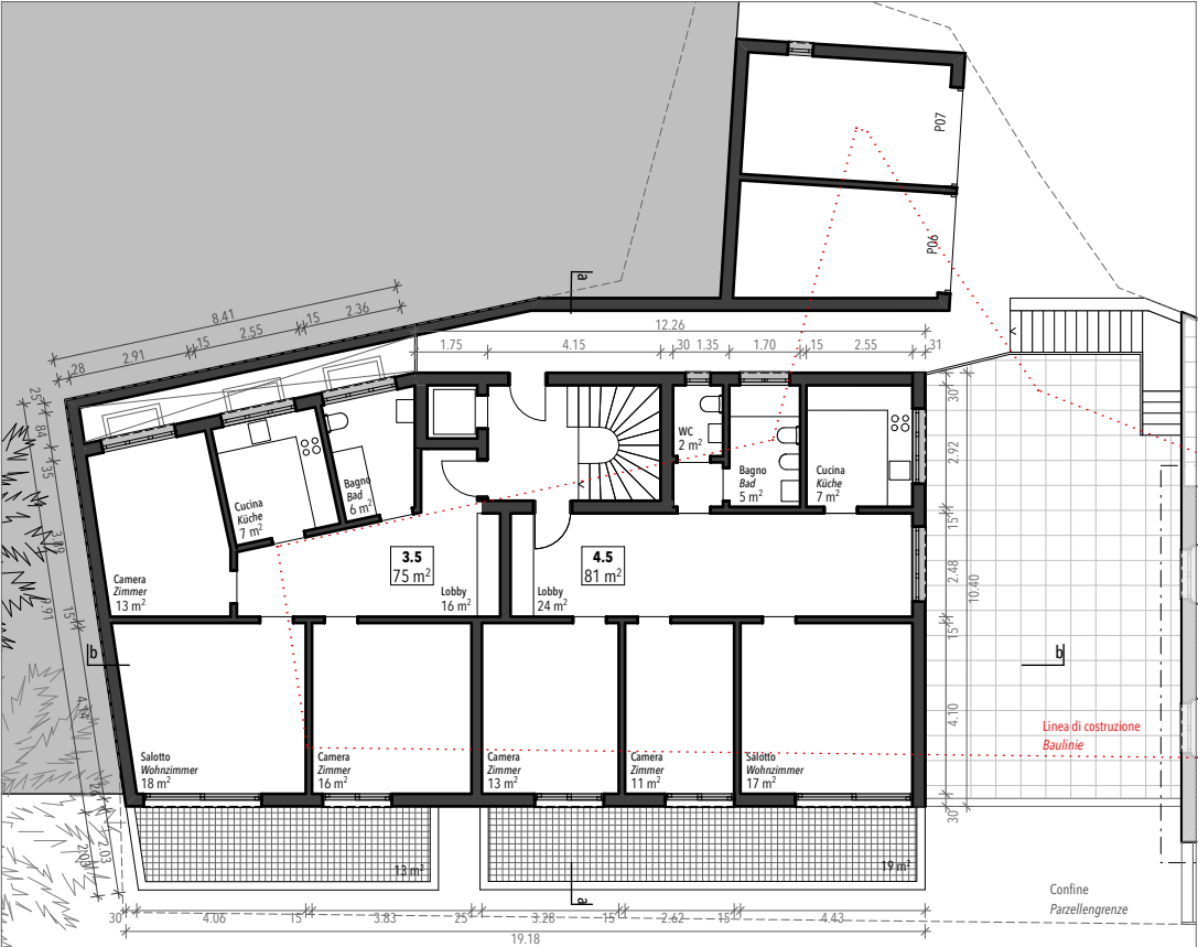
3. piano | 3. Obergeschoss
