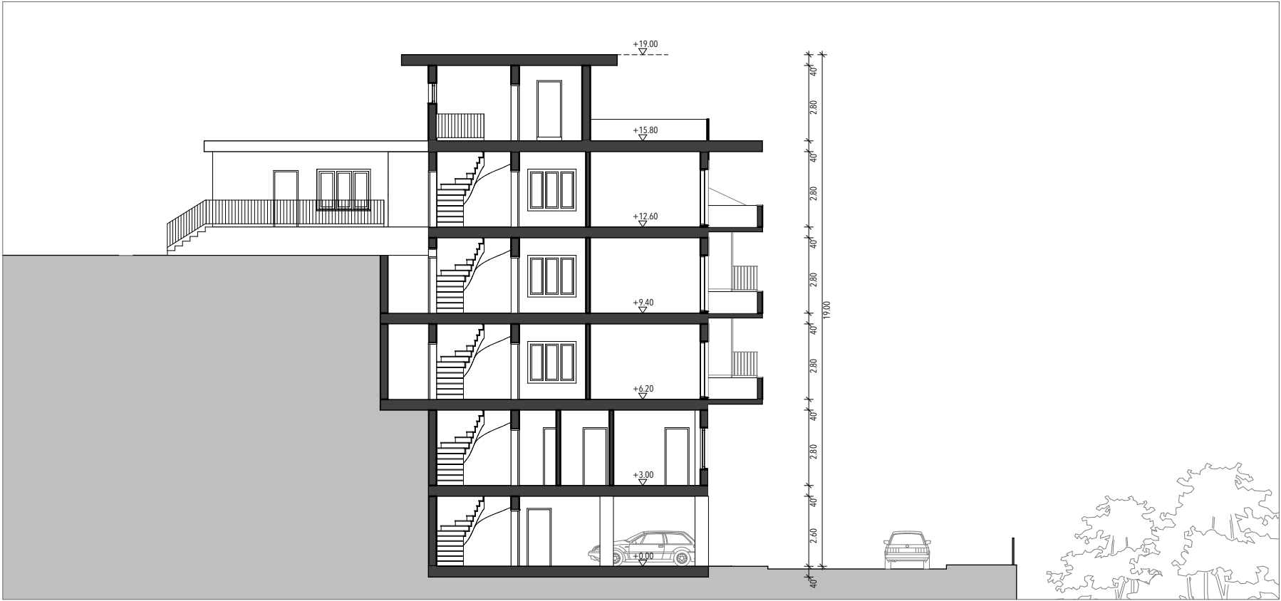
Sezione AA | Schnitt AA
