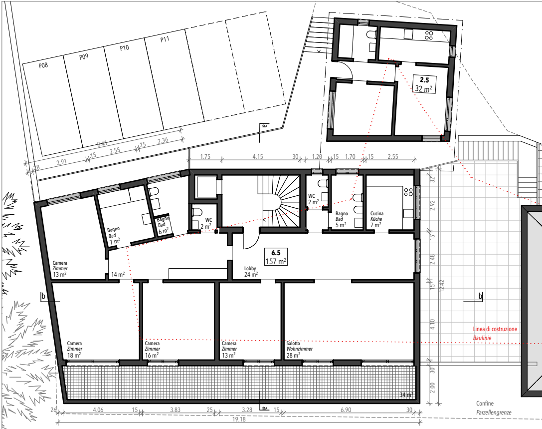
4. piano | 4. Obergeschoss
