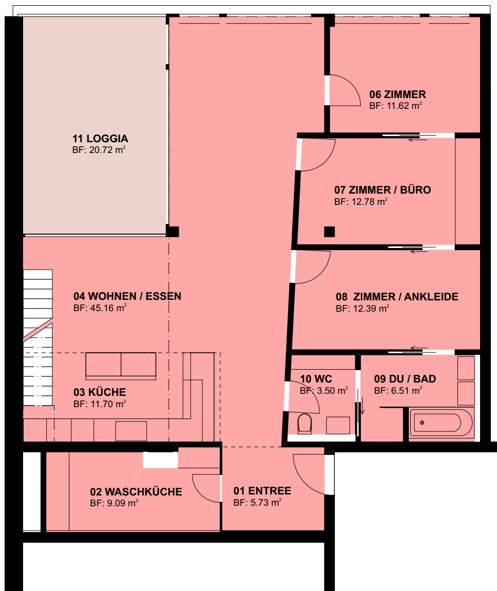
Grundriss Erdgeschoss Mst.1:100
