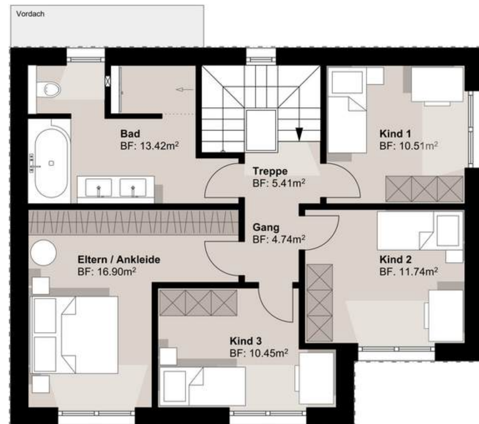
Haus Nr. 03, 08 Grundriss OG, (6.5 Zimmer EFH) Brutto-Geschossfläche = 92.30m 2 1:100
