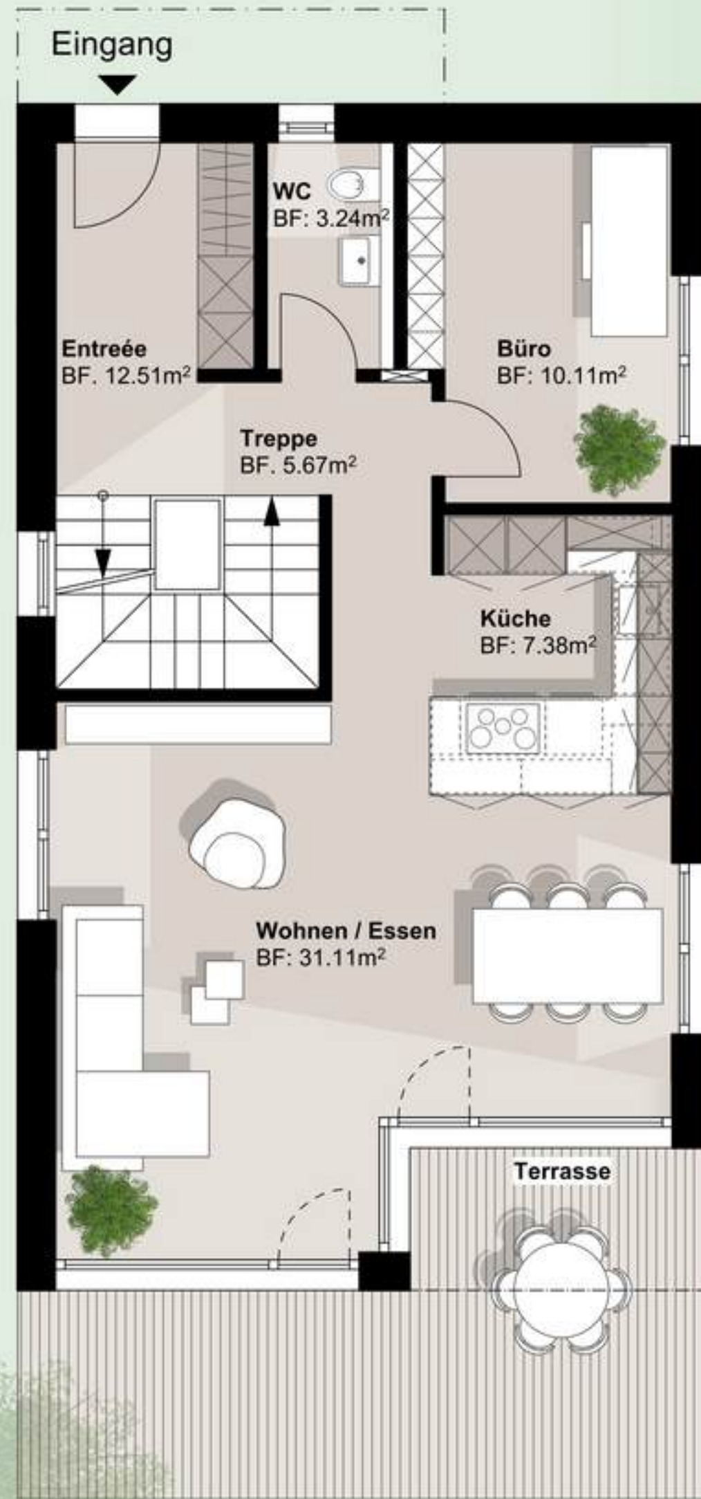
Haus Nr. 07, 11, 12 Grundriss EG (5.5 Zimmer EFH) Brutto-Geschossfläche = 86.50m 2 + Terrasse 20.81m 2 1:100
