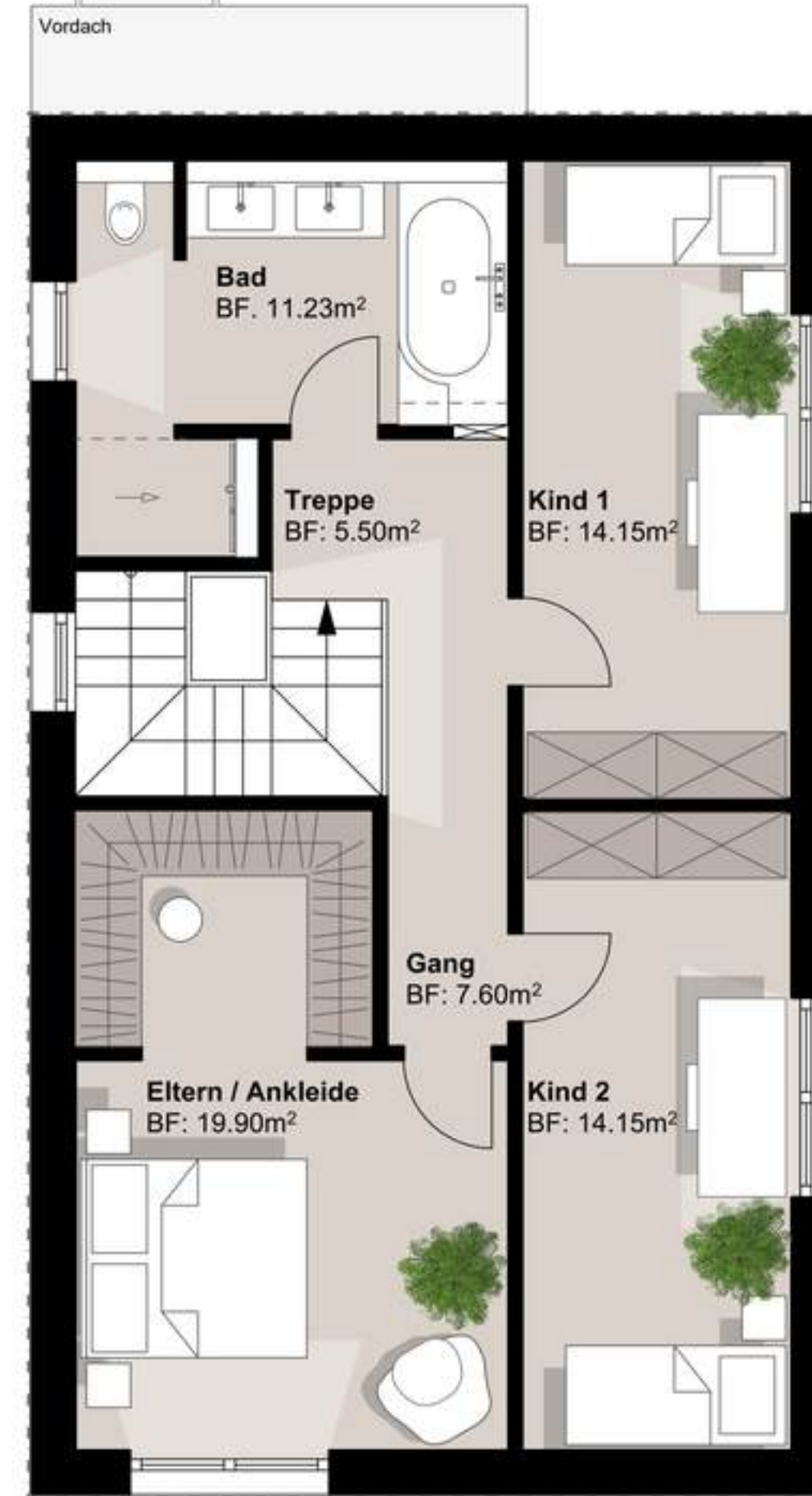
Haus Nr. 16 Grundriss OG, (5.5 Zimmer EFH) Brutto-Geschossfläche = 91.25m 2 1:100
