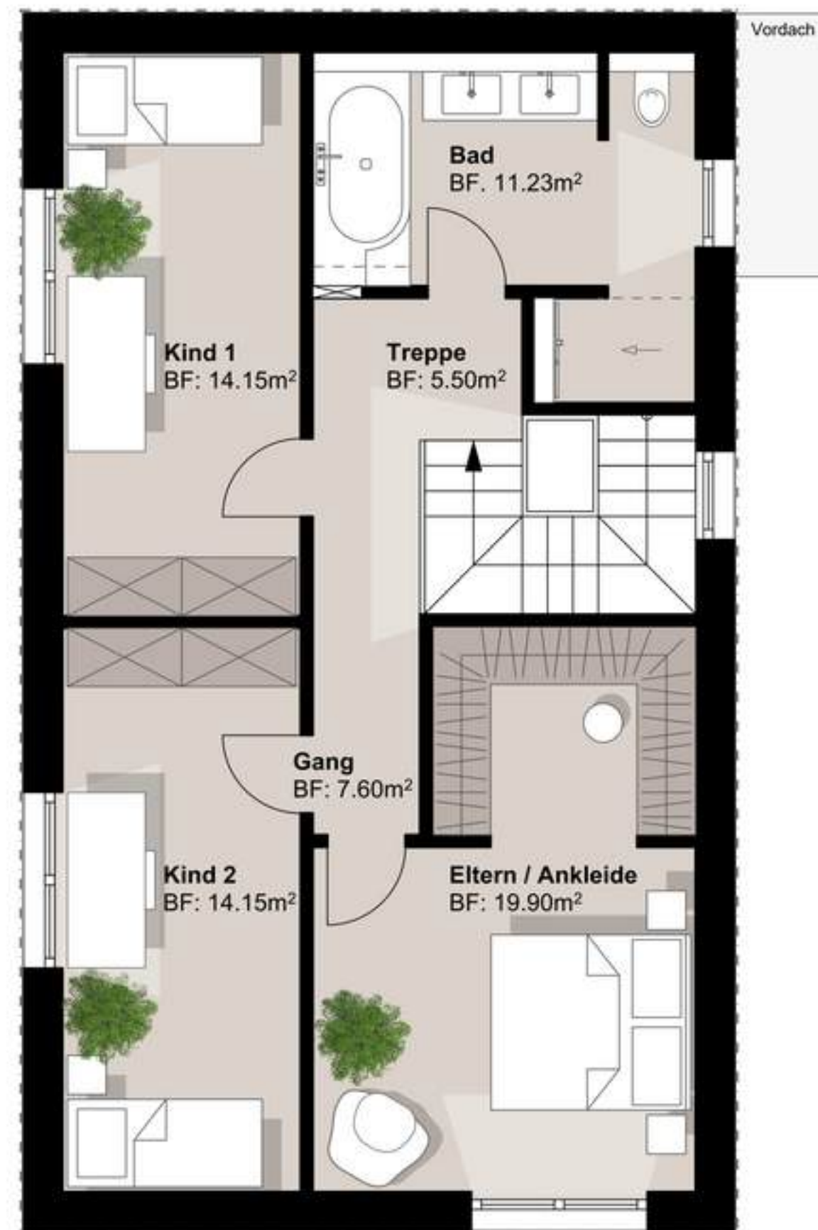
Haus Nr. 14 Grundriss OG, (5.5 Zimmer EFH) Brutto-Geschossfläche = 91.25m 2 1:100
