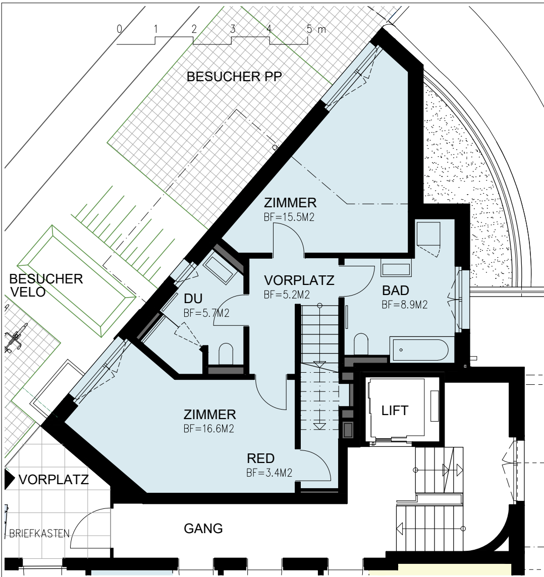
ERDGESCHOSS
