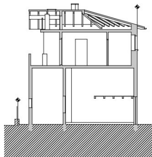
SEZIONE S01
