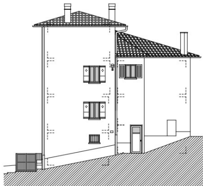
PROSPETTO EST
