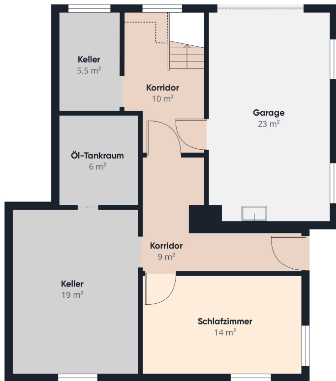
Etage 0
