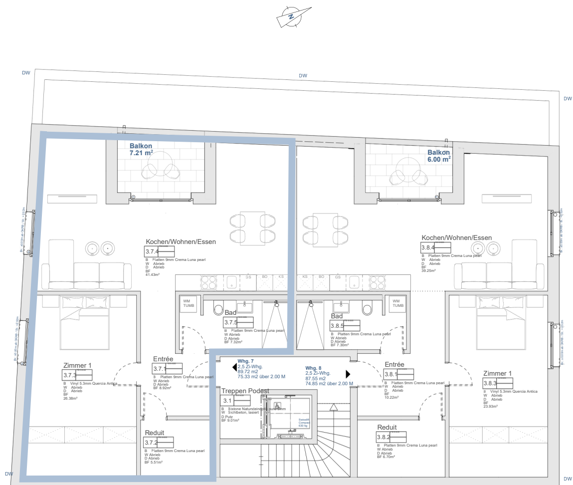
GRUNDRISS DACHGESCHOSS 1:100
