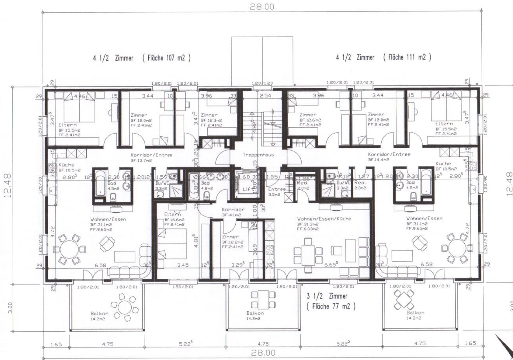
Grundriss 1.0bergeschoss Spinsstrasse 2E (nicht Massstab getreu)
