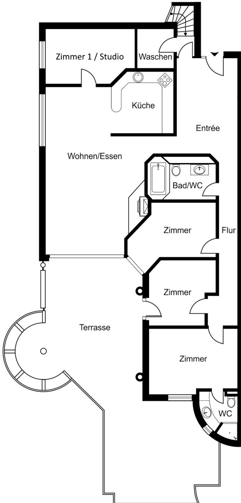
2. Obergeschoss
