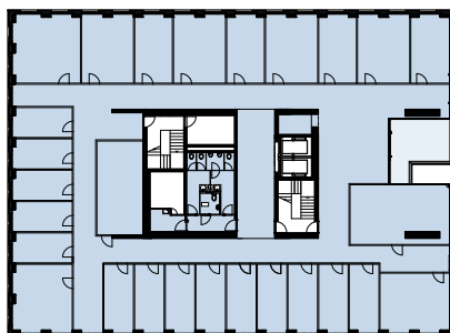
3. OBERGESCHOSS Nutzfläche: 879.2 m 2
