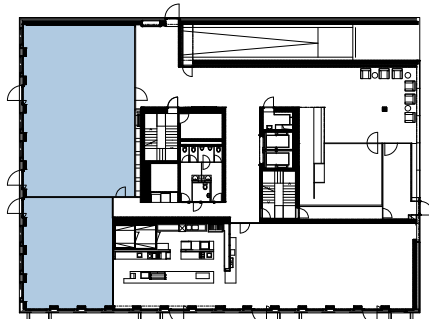
ERDGESCHOSS Nutzfläche: 264.8 m 2
