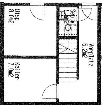
Untergeschoss
