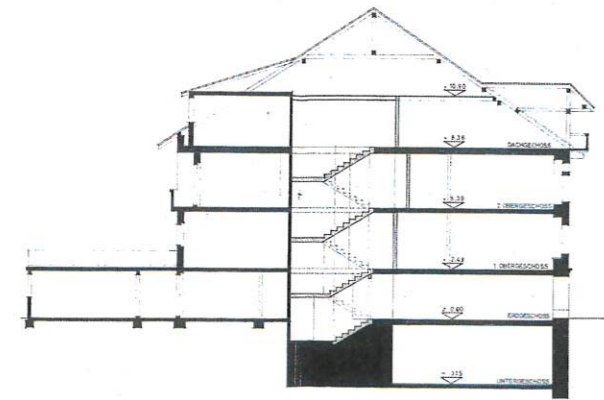
Schemaschnitt
