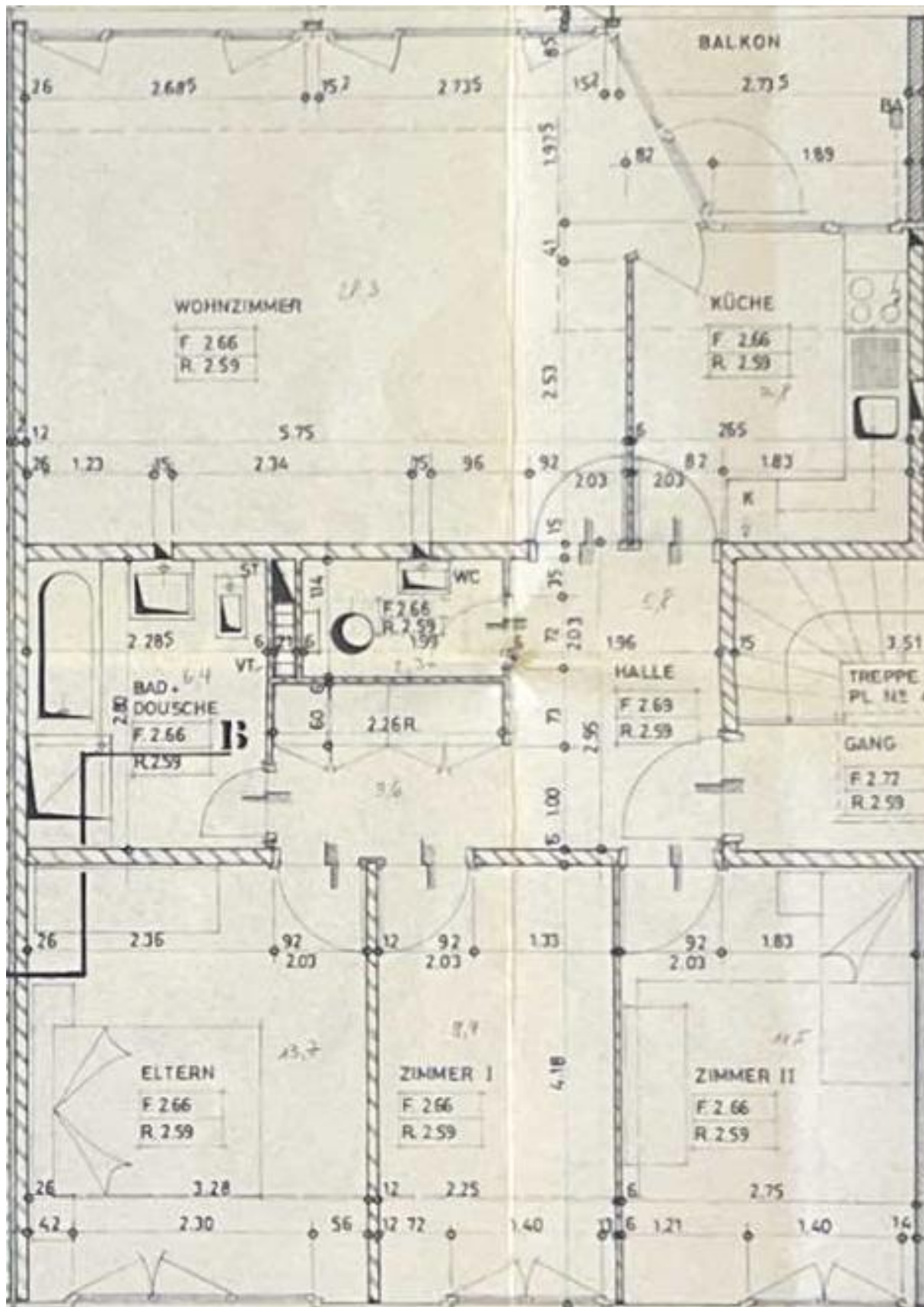
Beundenring 33 / 35, Nidau Grundriss 4.5-Zimmerwohnung links
