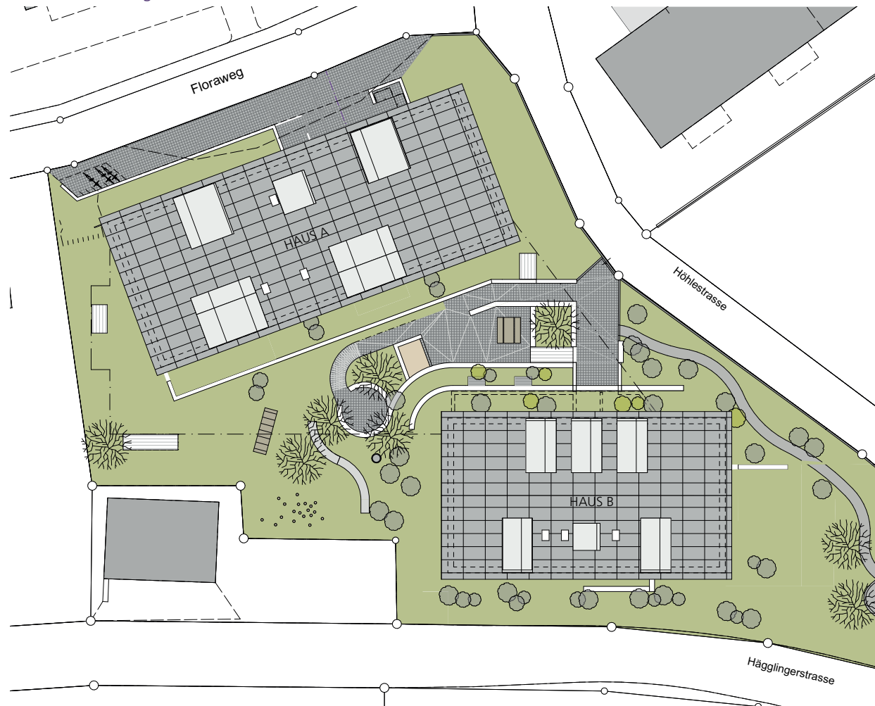
Photovoltaikanlage auf Dächer FloraPark
