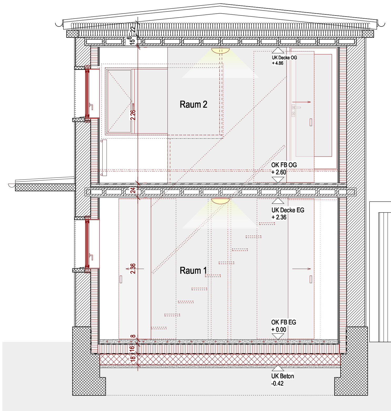
Querschnitt Räume 1 : 33
