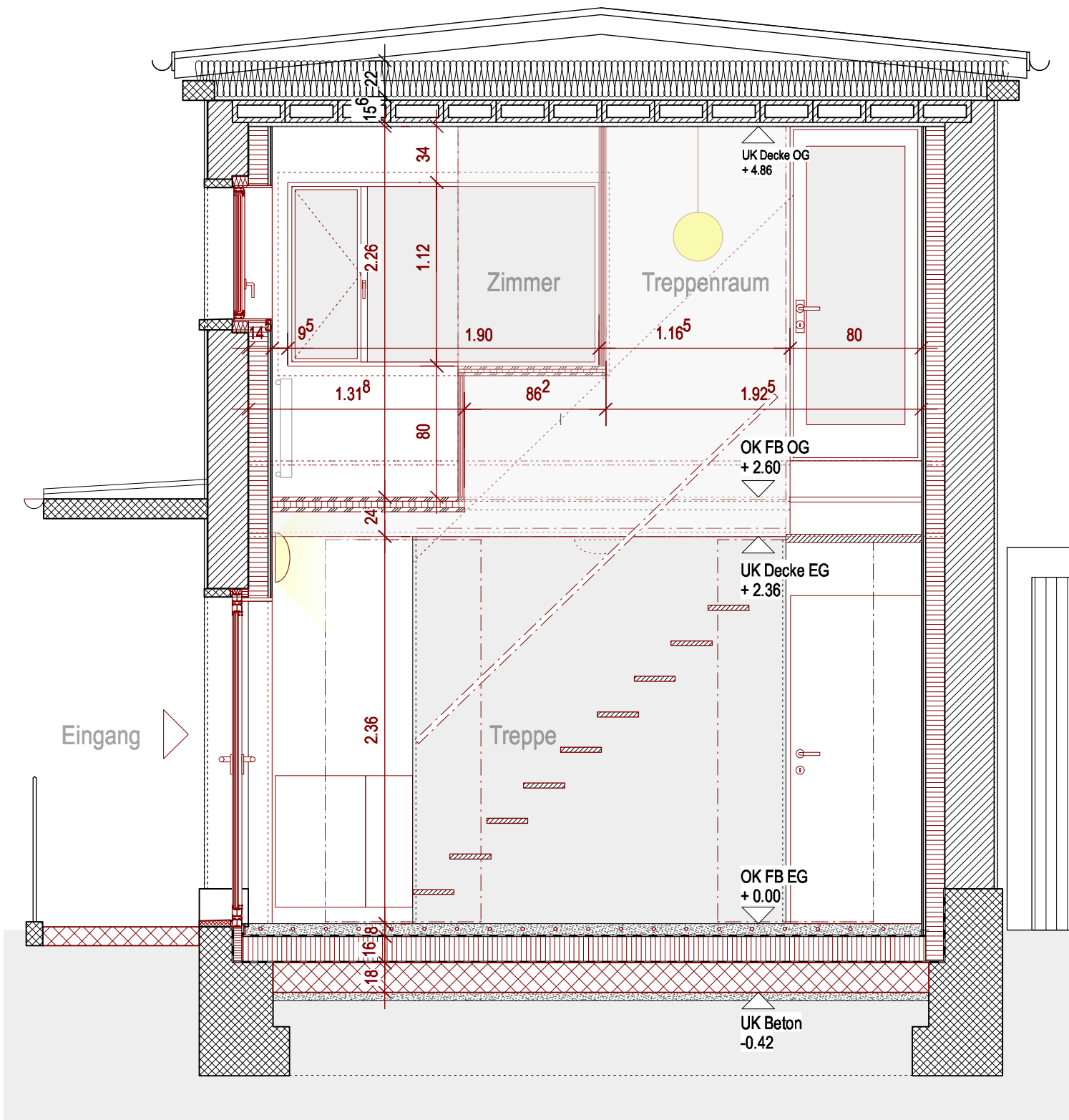
Querschnitt Treppe 1 : 33
