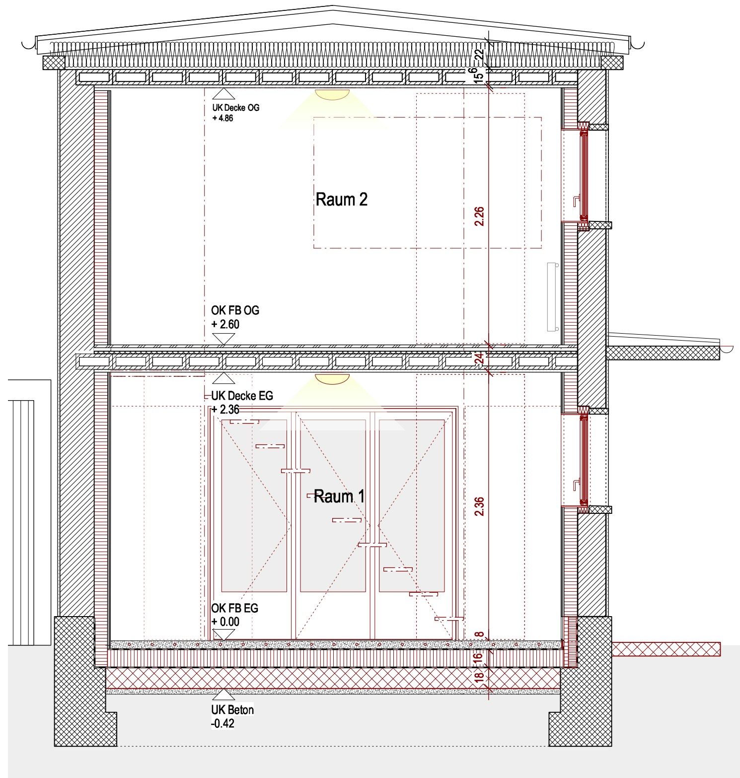
Querschnitt Räume 1 : 33 Blickrichtung Schwalbenweg
