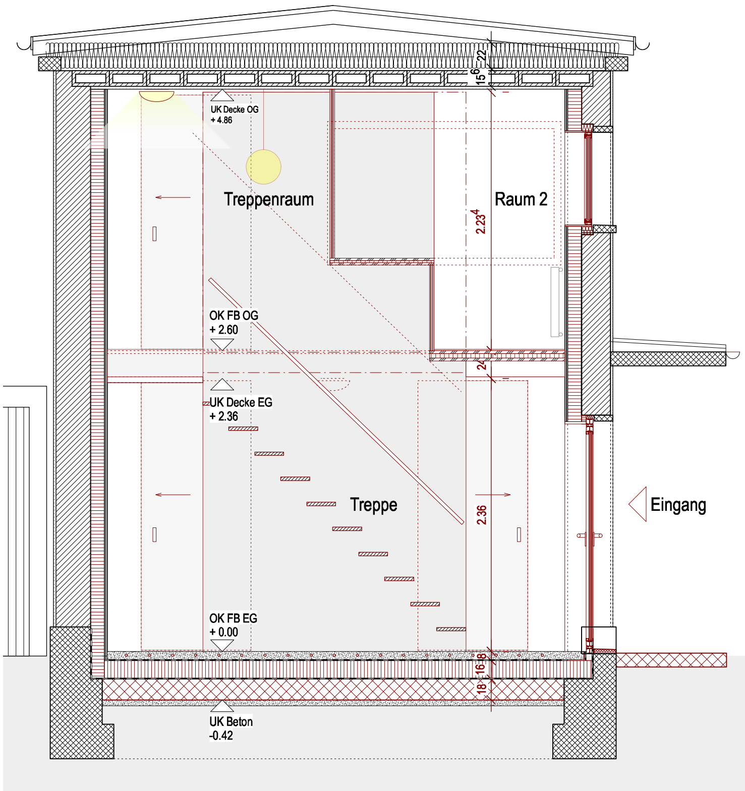
Querschnitt Treppe 1 : 33 Blickrichtung Schwalbenweg
