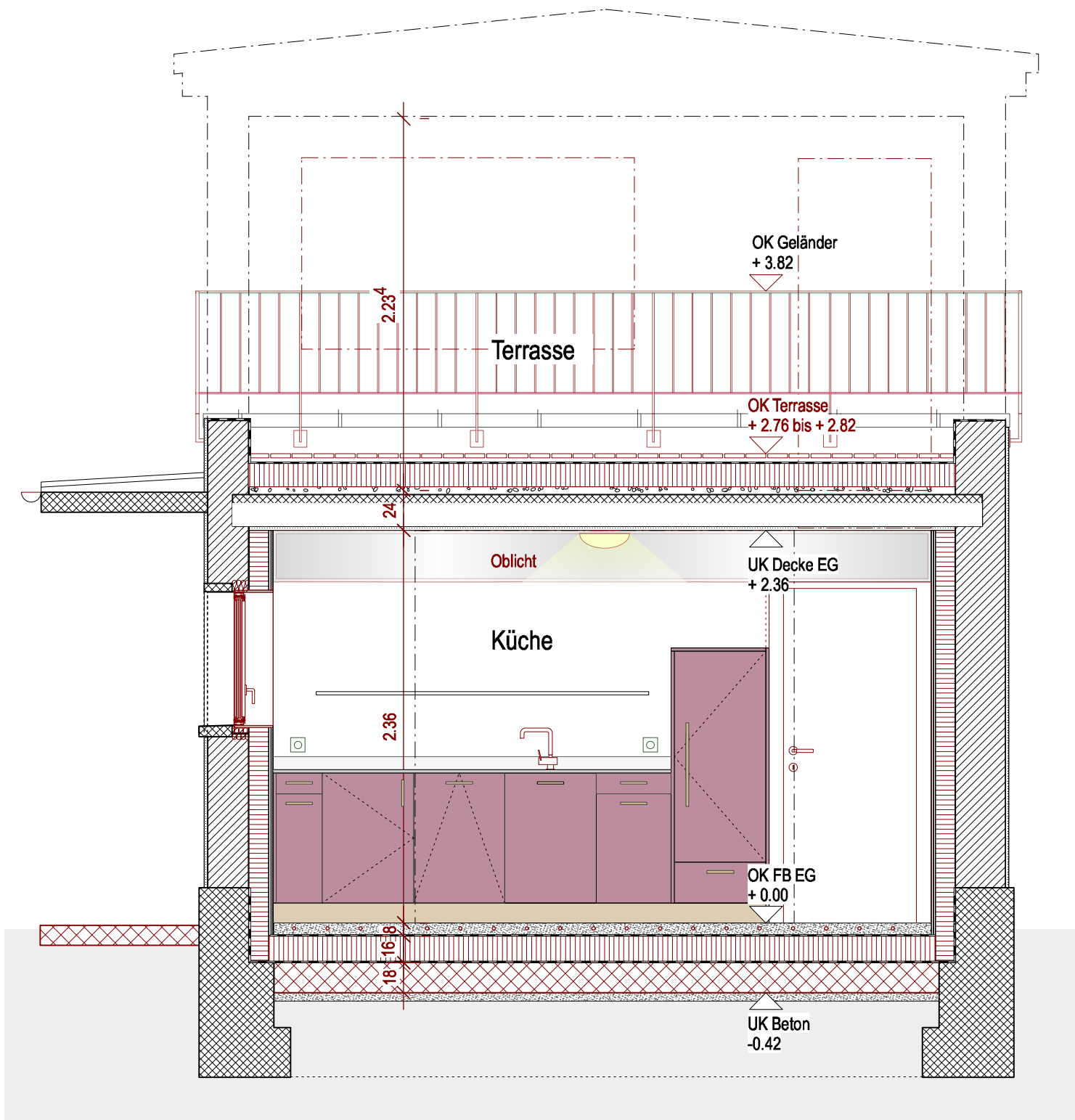
Querschnitt Küche 1 : 33
