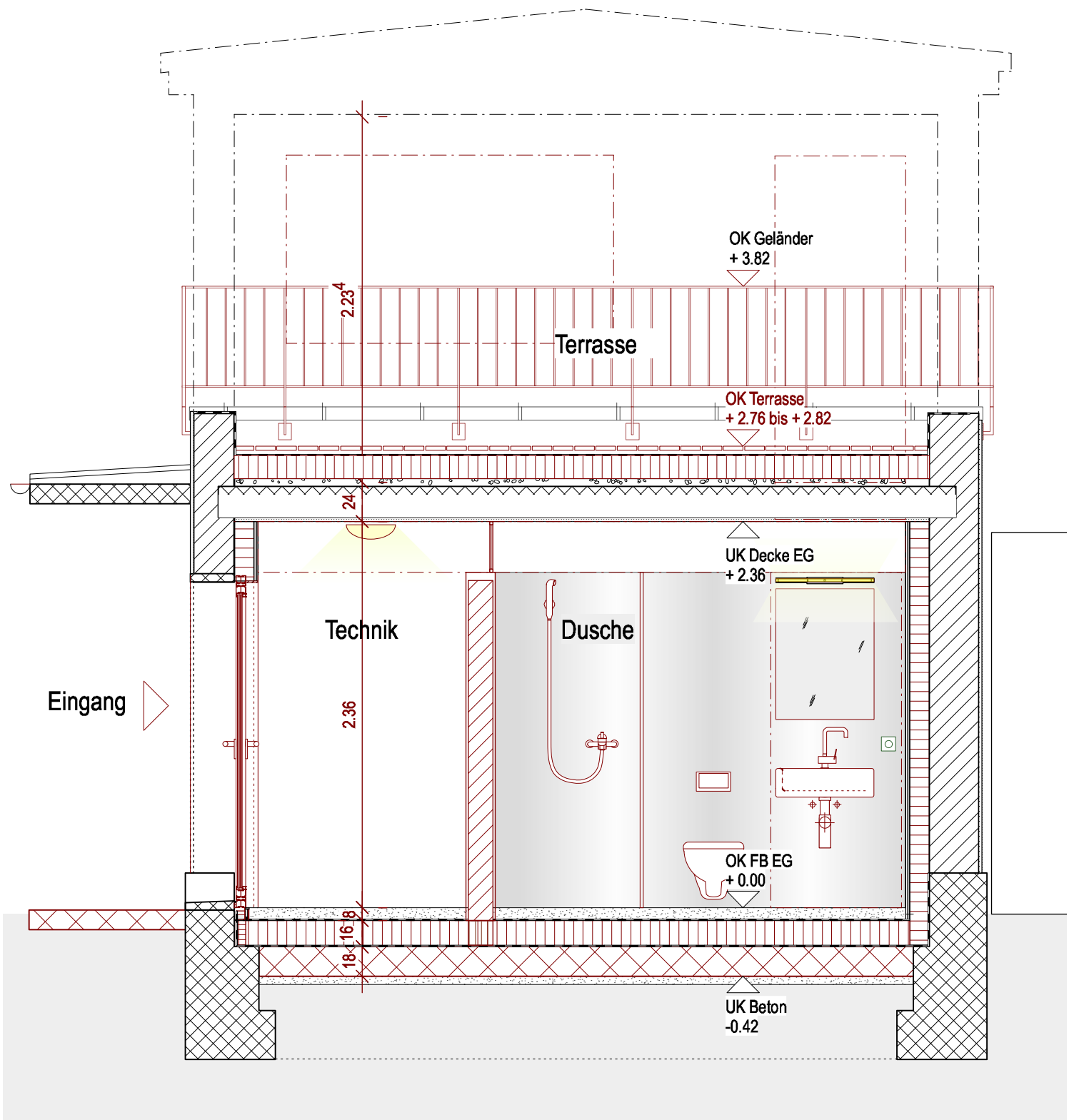
Querschnitt Dusche 1 : 33
