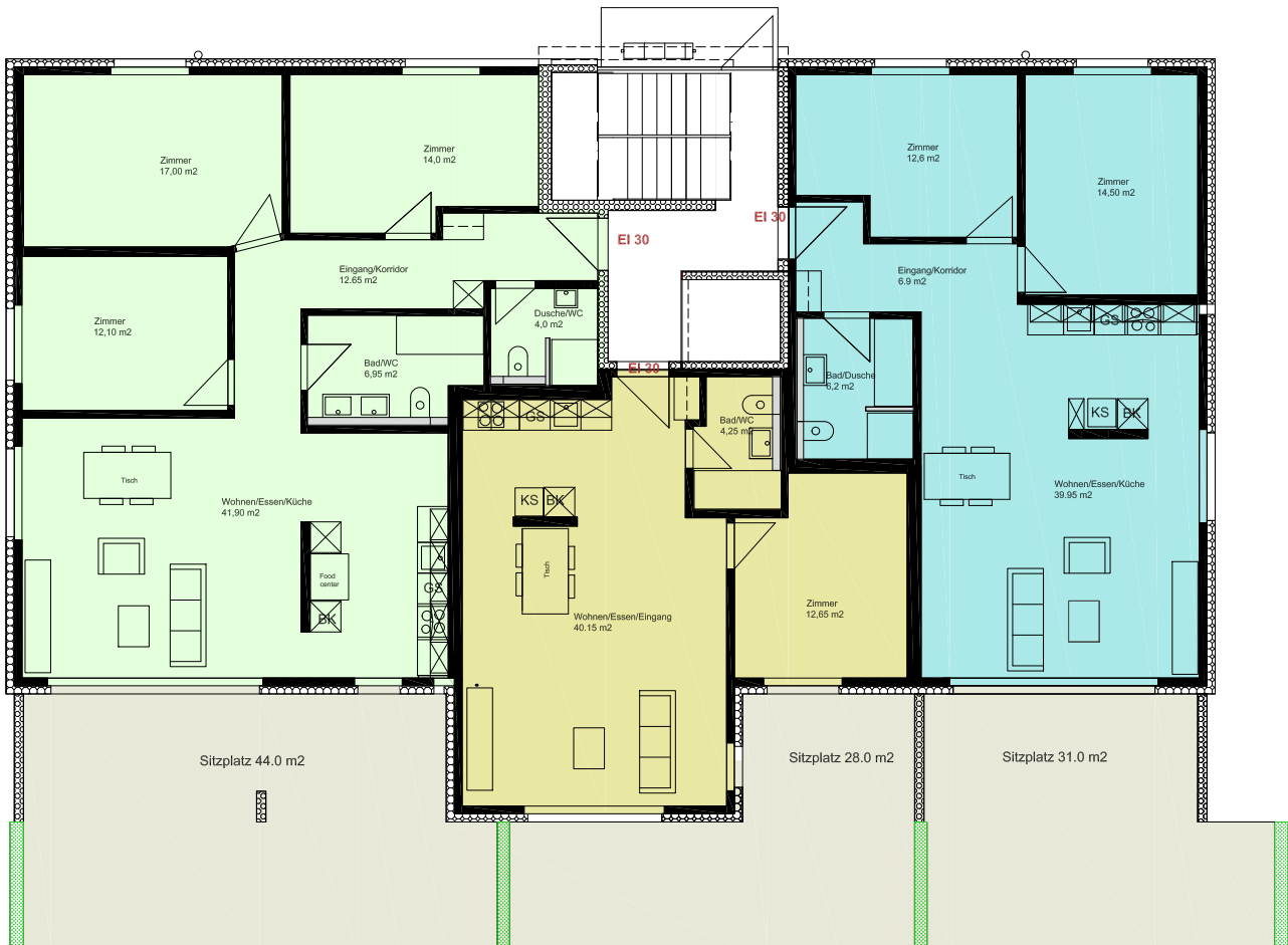
4 1/2-Zimmerwohnung BGF 123,95 m 2
