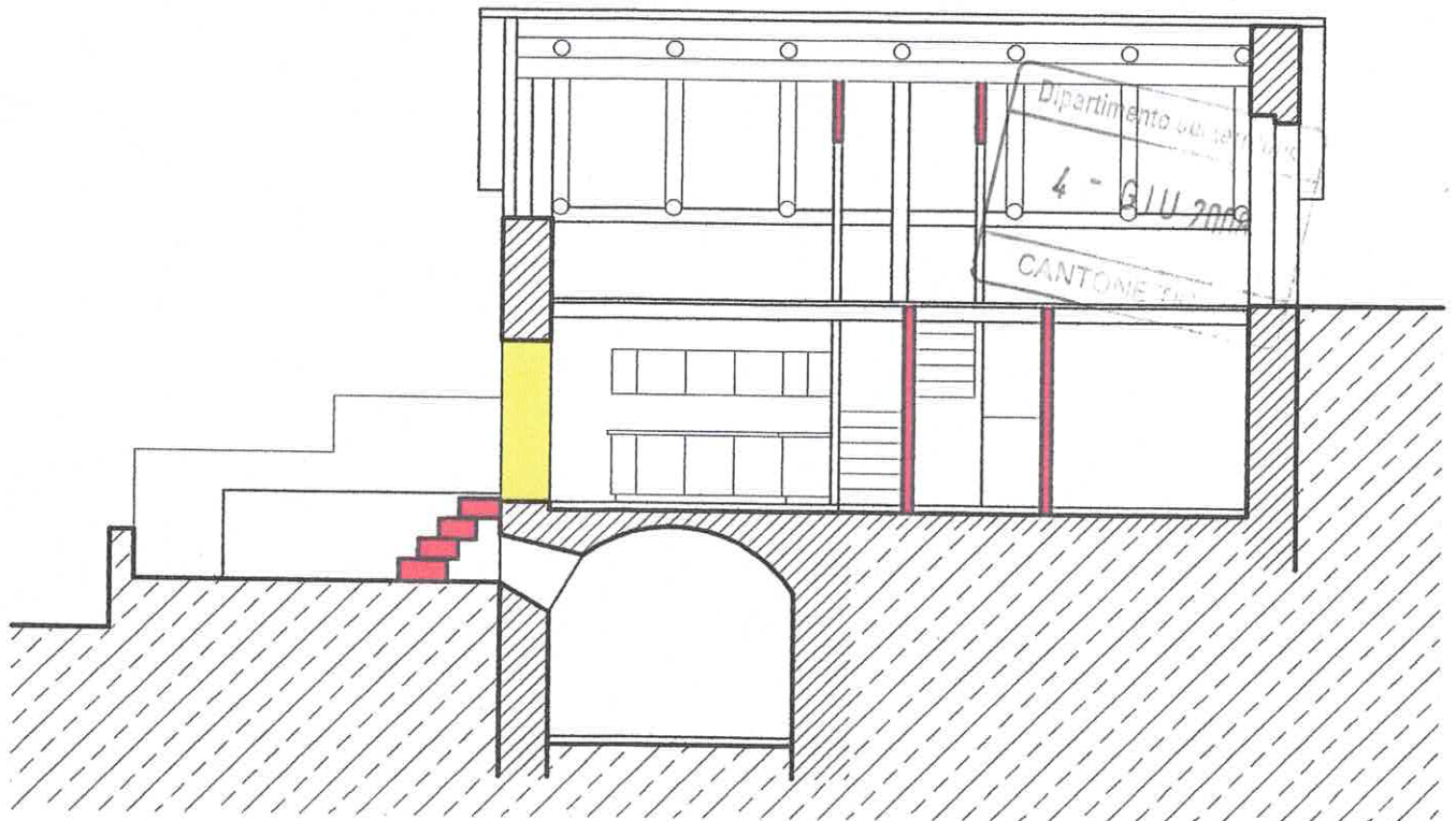
SEZIONE TRASVERSALE
