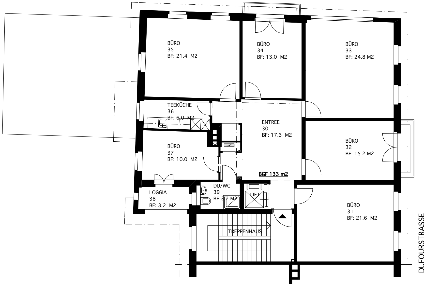
GESCHÄFTSHAUS DUFOURSTRASSE 147, 8008 ZÜRICH GRUNDRISS 3.OBERGESCHOSS
