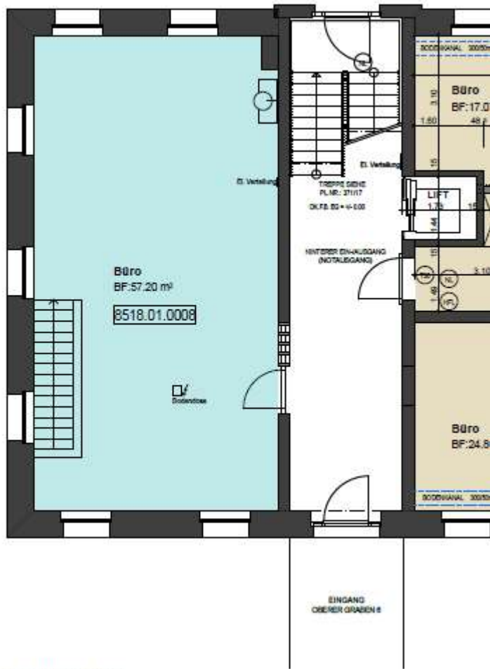
ERDGESCHOSS
