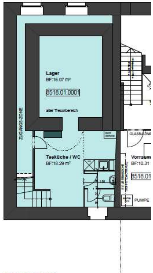
UNTERGESCHOSS
