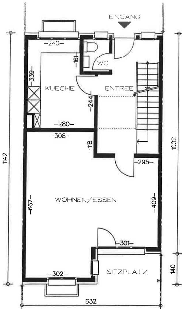
ERDGESCHOSS
