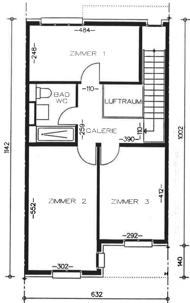
1. OBERGESCHOSS
