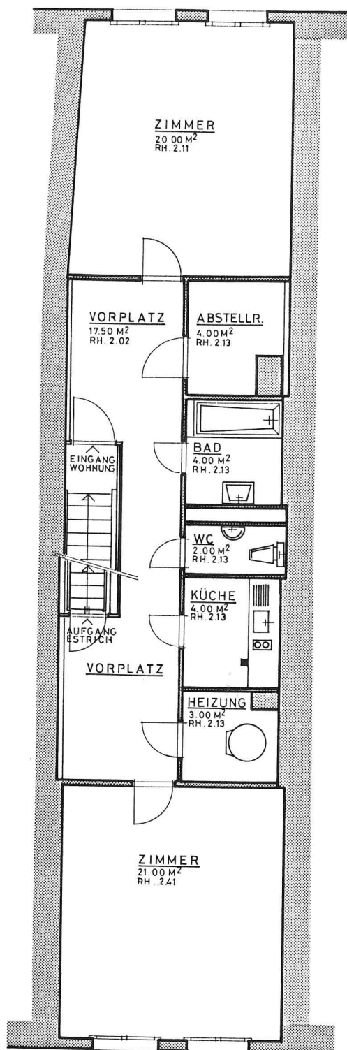
4. OBERGESCHOSS
